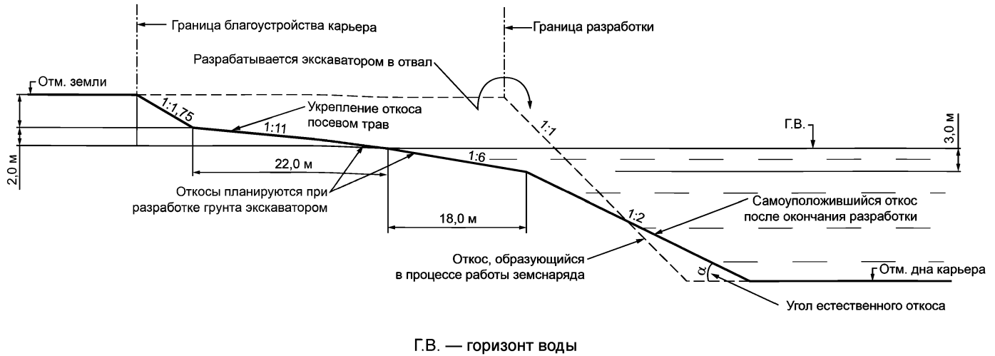
Рисунок К.1 — Водоем для объектов рыбохозяйственного производства
