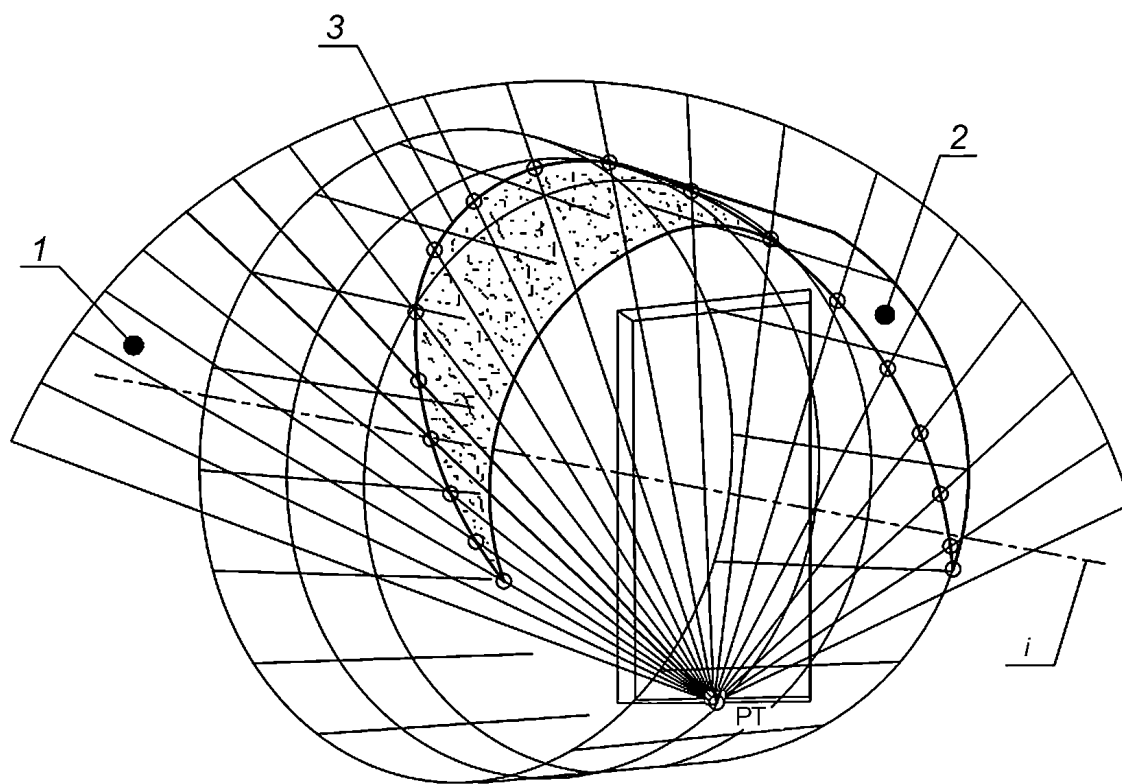
1 — суточный конус солнечных лучей; 2 — солнцезащитное устройство; 3 — контур СЗУ; i — ось цилиндра
