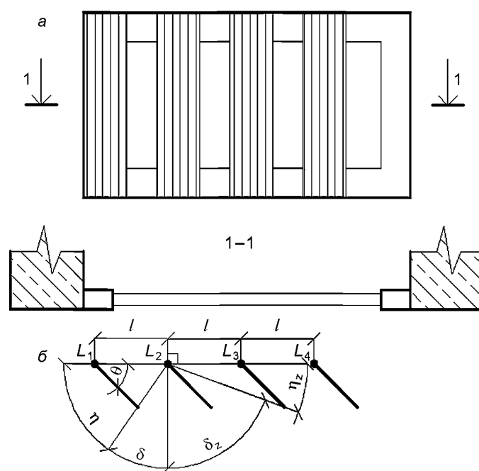
а — фасад; б — разрез 1—1
