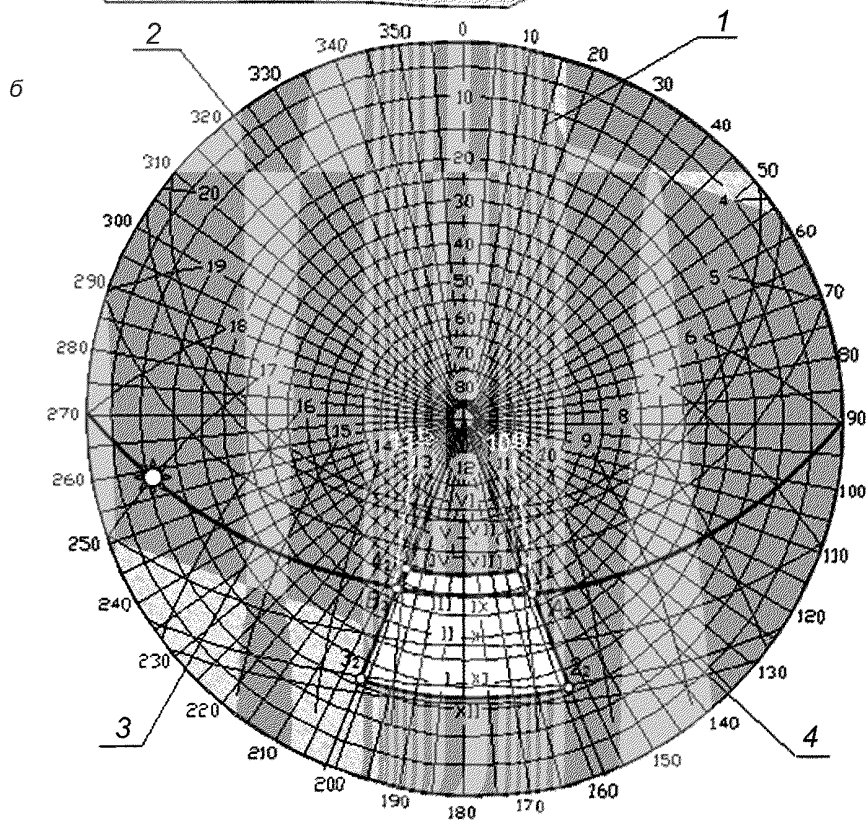
а — построение теневой маски; б — солнечная карта
