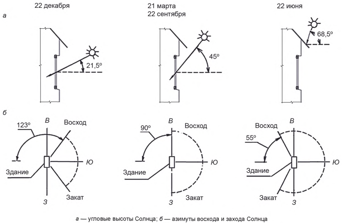
Рисунок 2 — Солнечные углы для фасада южной ориентации (45° с. ш.)
