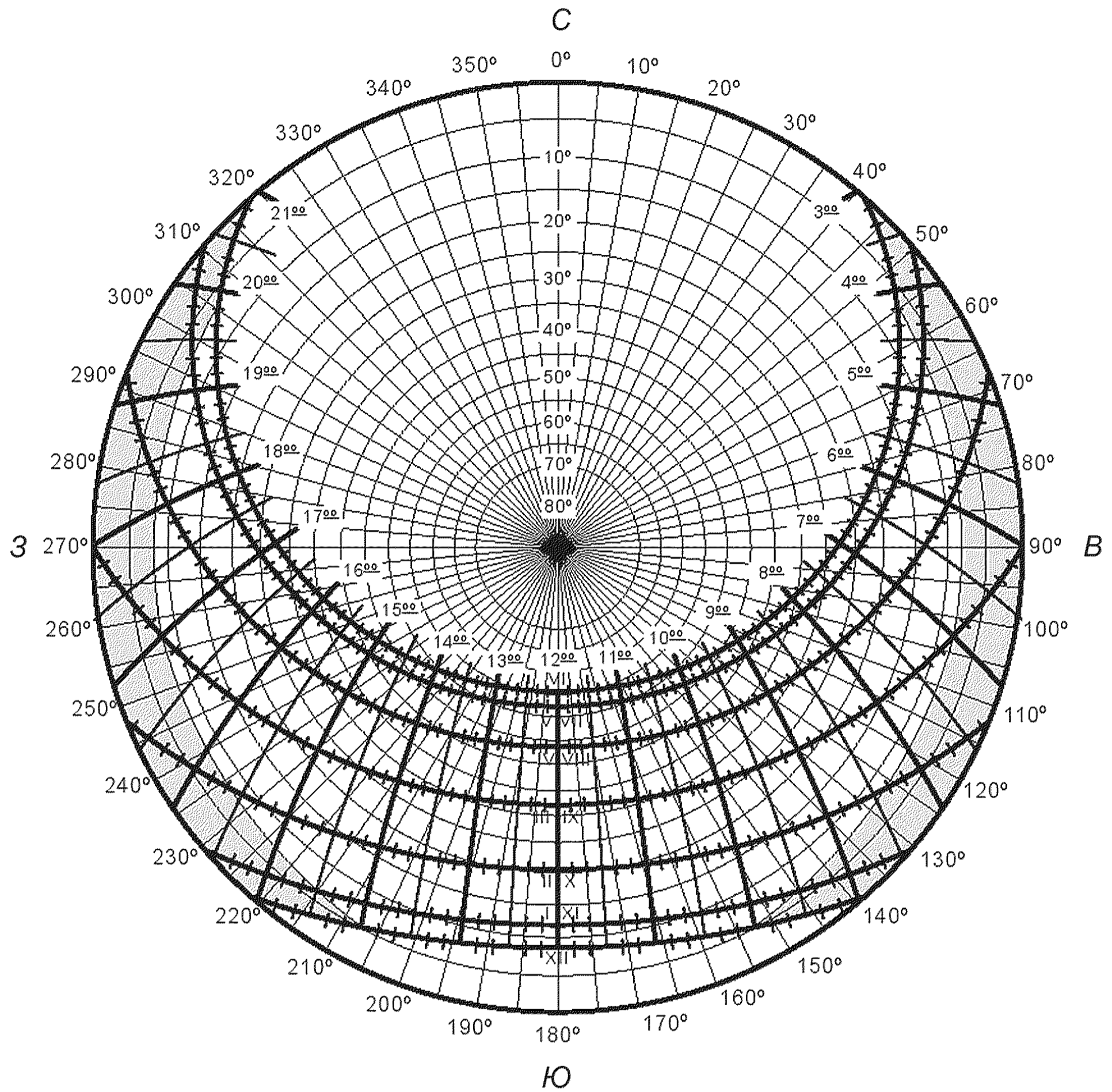
Рисунок К.10 — Солнечная карта для 58° с. ш.
