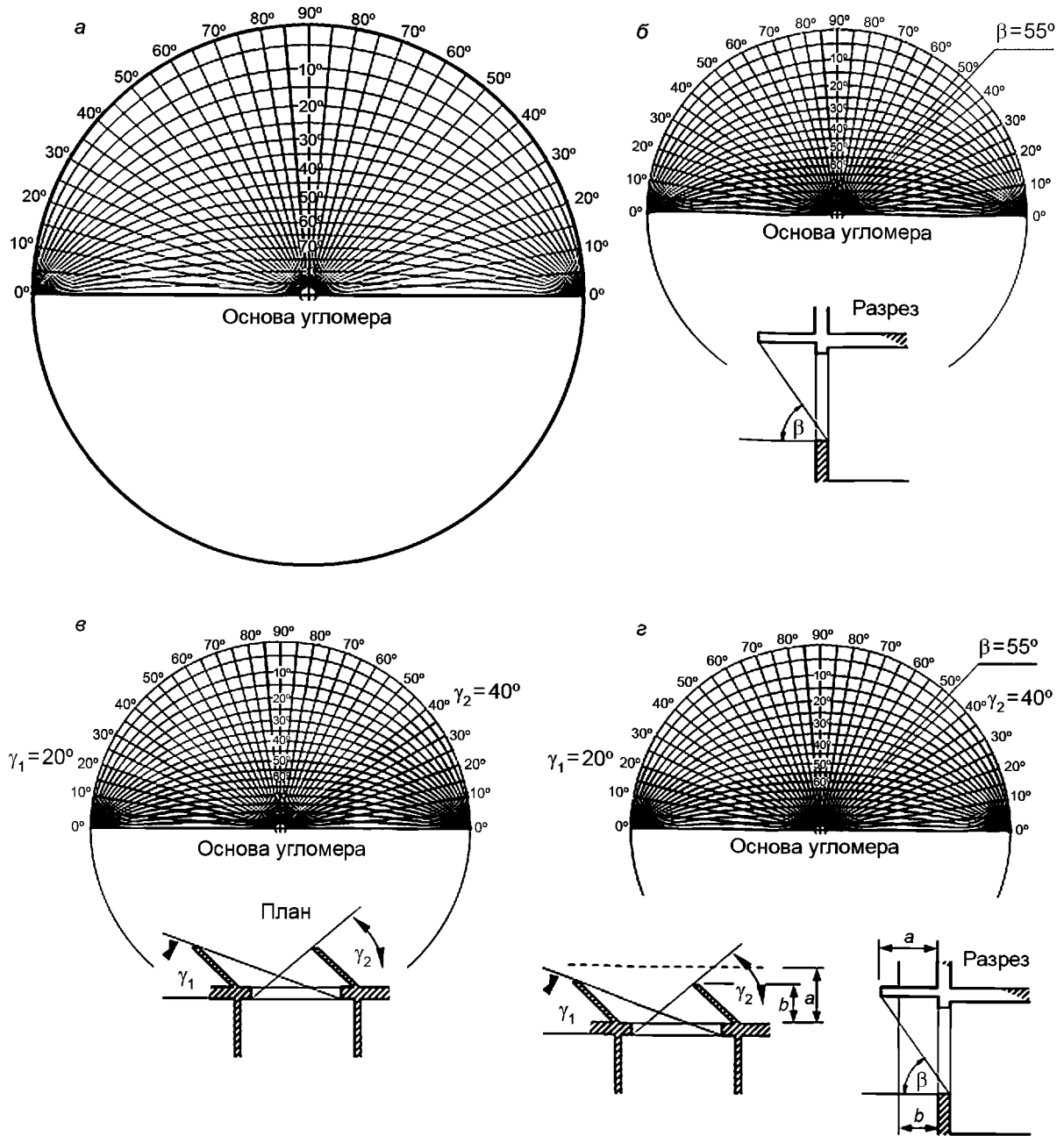
а — теневого угла; б — теньевая маска горизонтального СЗУ; в — теньевая маска вертикального СЗУ; г — теньевая маска комбинированного СЗУ
