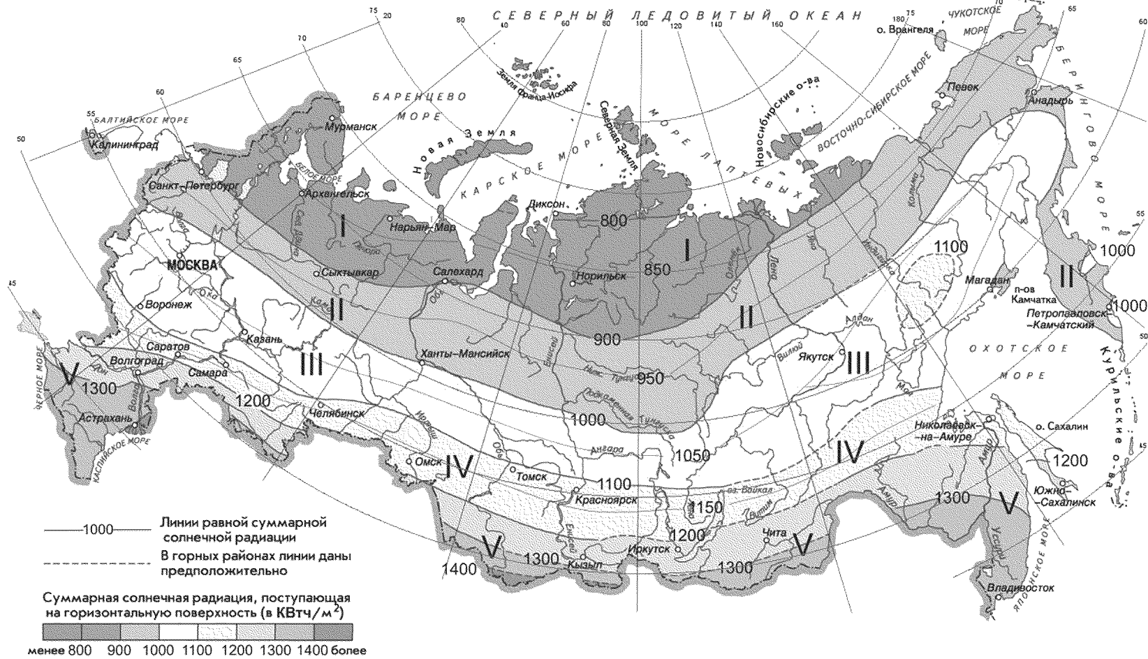
Рисунок А.1 — Схематическая карта суммарной годовой солнечной радиации на горизонтальную поверхность в условиях действительной облачности, кВт·ч/м 2
