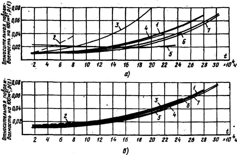
Рис. П1.7. Текущие кривые вероятности аварийного пробоя микалентной изоляции генераторов наблюдаемой совокупности, работающей в воздушной среде:
