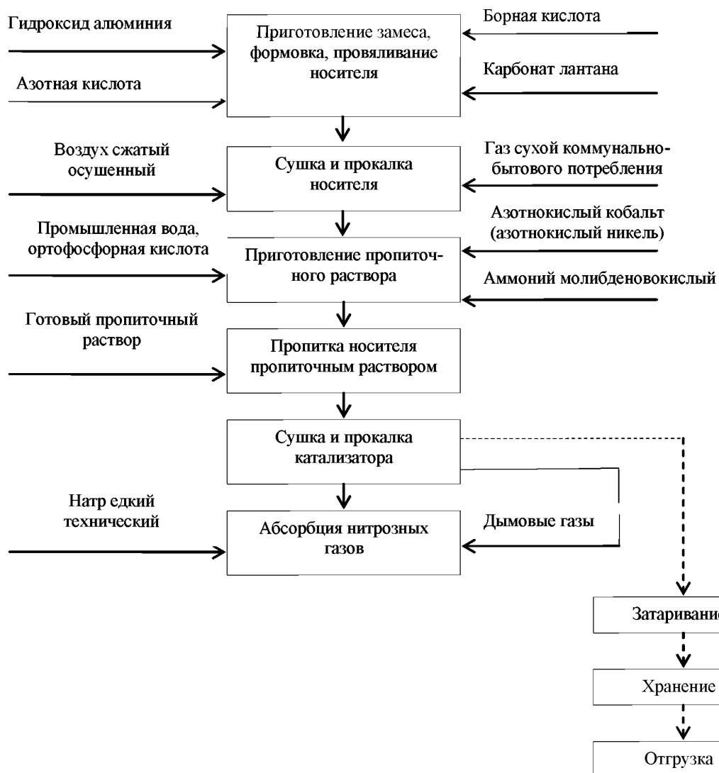
Рисунок 5.9 — Схема производства алюмоникелькобальтмолибденовых катализаторов
