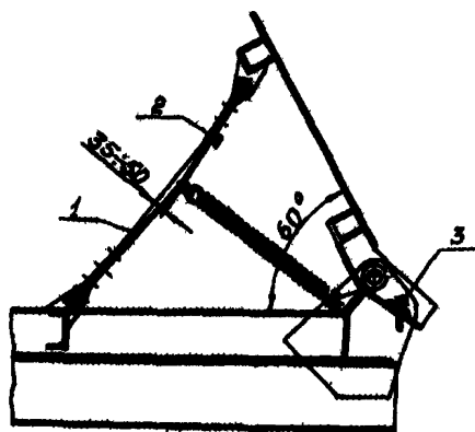
1-трос; 2-зажим; 3-стопорный палец.
