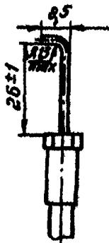
Трос переключения крана управления делителем.
