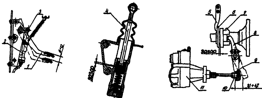
Регулировка свободного хода педали сцепления.
