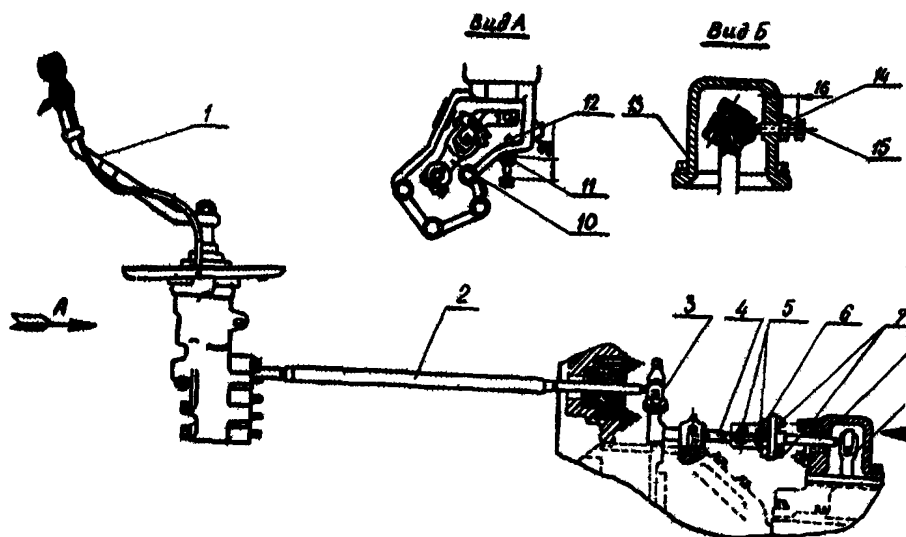
Привод управления механизмом переключения передач.
