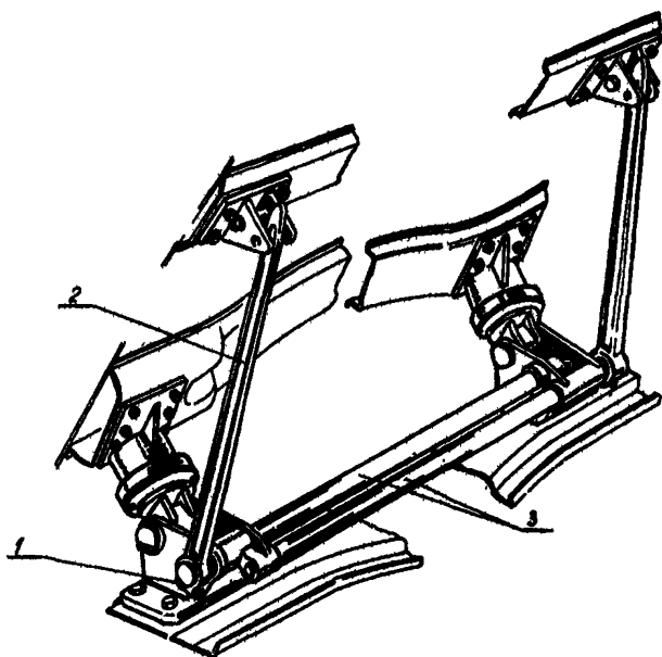
1-стяжной болт; 2-рычаг торсиона; 3-торсион.
