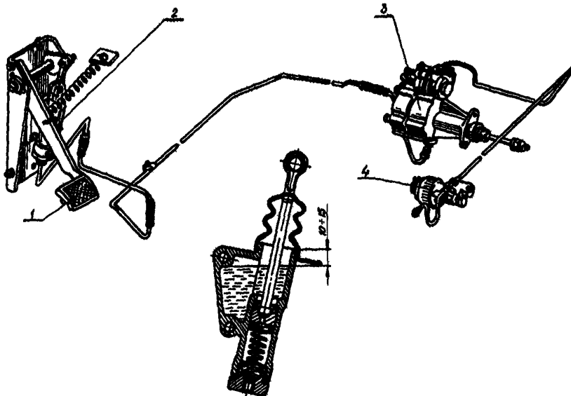
1-педадь сцепления; 2-главный цилиндр управления сцеплением; 3-пневмогидравлический усилитель; 4-редукционный клапан.
