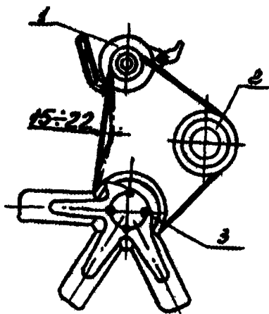
1-шкив генератора; 2-шкив насоса; 3-шкив коленчатого вала.
