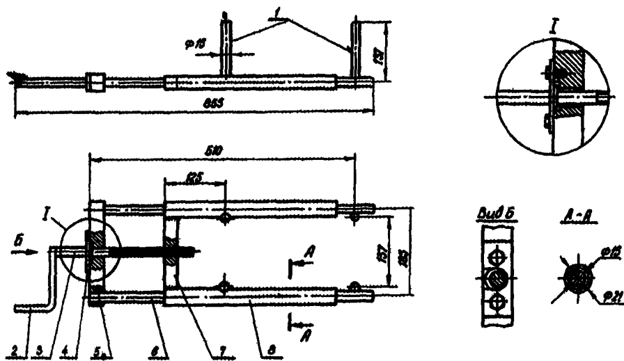
1-палец; 2-вороток; 3-винт; 4-пластина; 5, 7-поперечина; 6-стержень; 8-труба.
