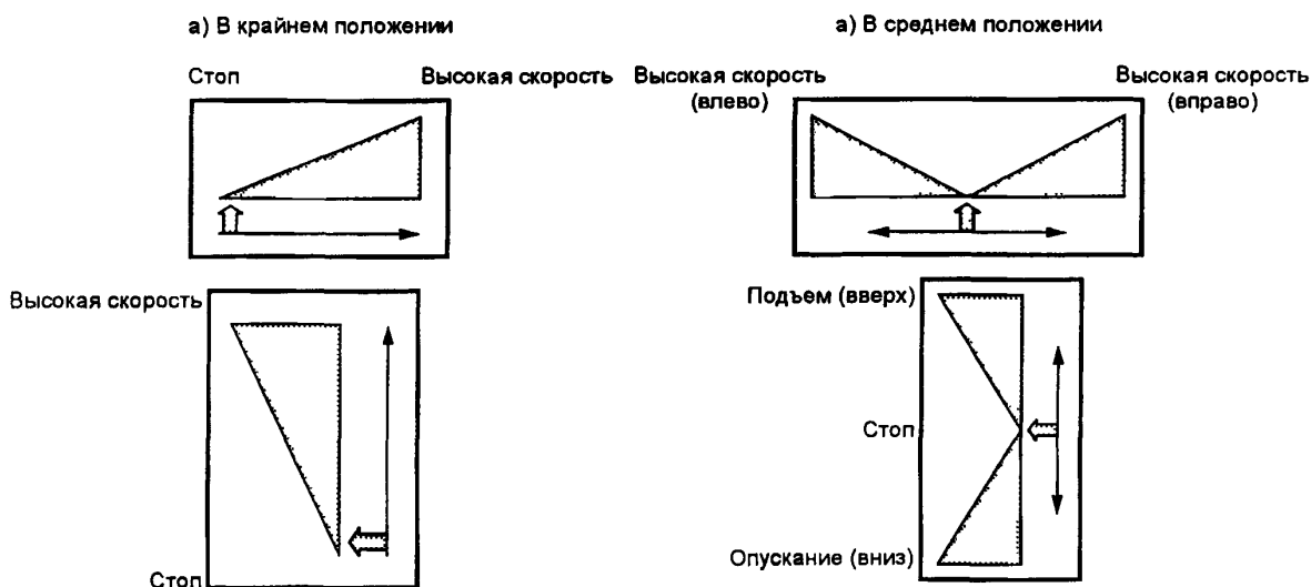
Рисунок 3 — Положение «СТОП» ползунка (пример линейного перемещения)
