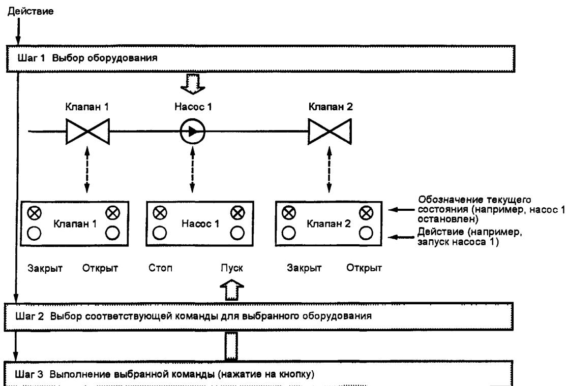
Рисунок 1 — Трехшаговая последовательность выполнения однофункционального применения
