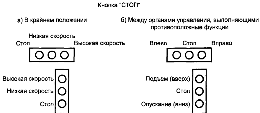
Рисунок 4 — Кнопка «СТОП» в наборе органов управления
