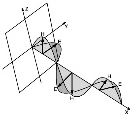
Рисунок 1 — Электромагнитное поле
