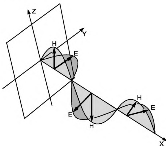
Рисунок 2 — Электромагнитное поле
