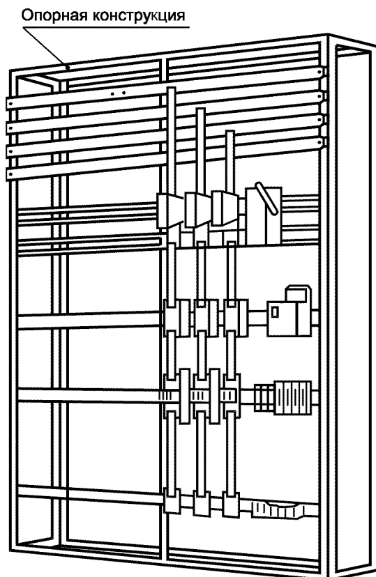
Рисунок С.1 — ИСУ заводского изготовления открытого типа
