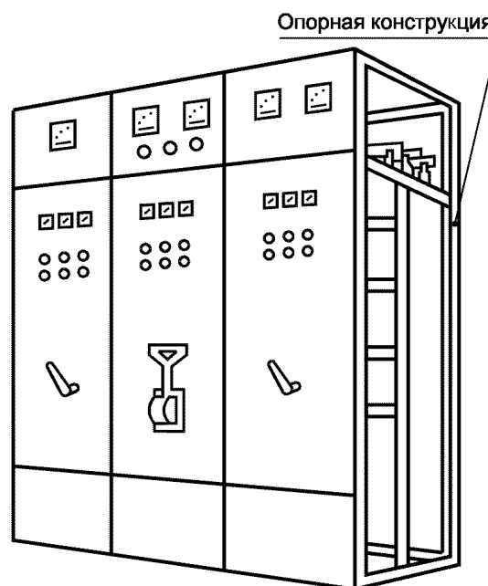
Рисунок С.2 — ИСУ заводского изготовления открытого типа, защищенное спереди
