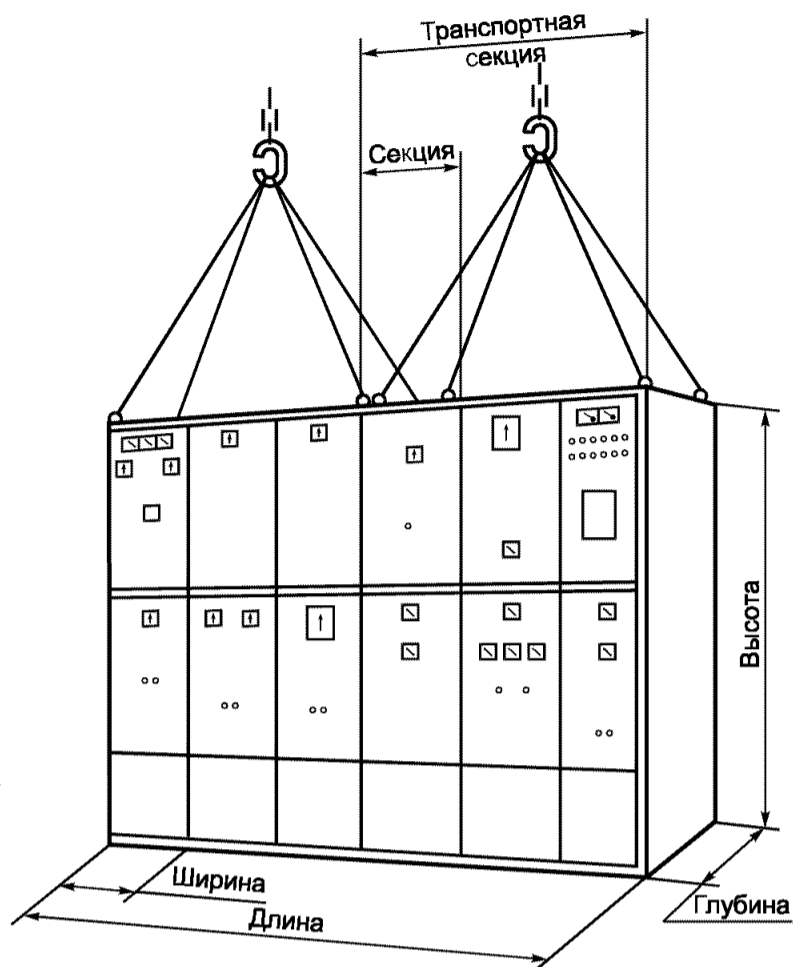
Рисунок С.4 — НКУ заводского изготовления много-шкафного типа
