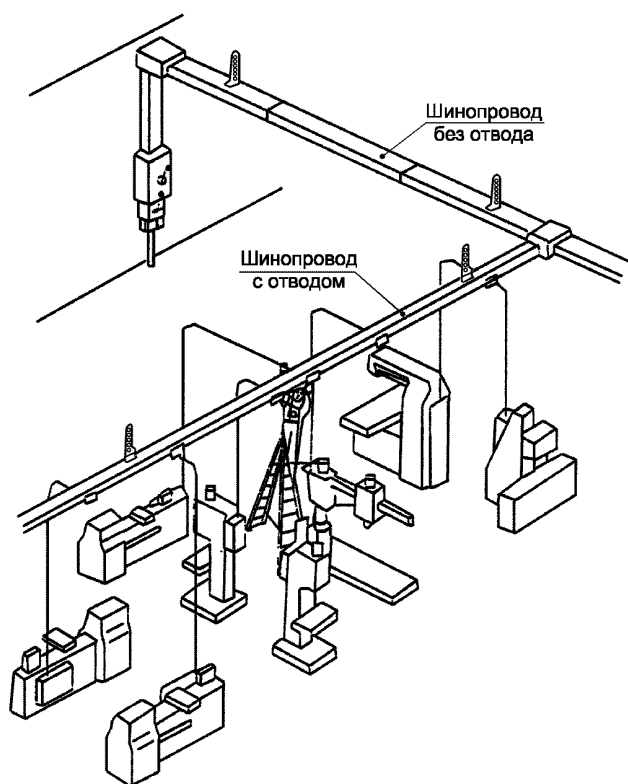
Рисунок С.7 — Система сборных шин (шинопровод)
