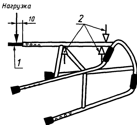
1 — заглушка; 2 — упоры
