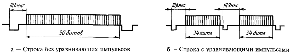
Рисунок 3 — Сигналы цифровых данных при тактовой частоте 1,734375 МГц
