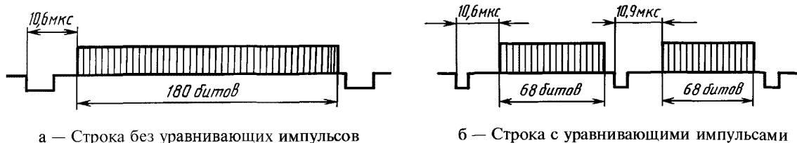
Рисунок 4 — Сигналы цифровых данных при тактовой частоте 3,468750 МГц
