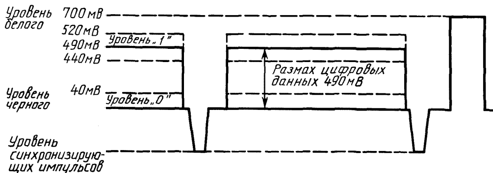
Рисунок 2 — Диаграмма уровней сигналов цифровых данных
