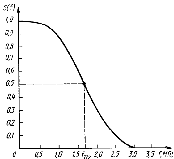
б — Спектральная плотность импульса при f_{T2} = 3,468750 МГц
