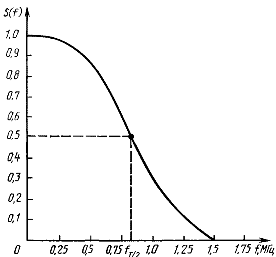
а — Спектральная плотность импульса при f_{T1} = 1,734375 МГц
