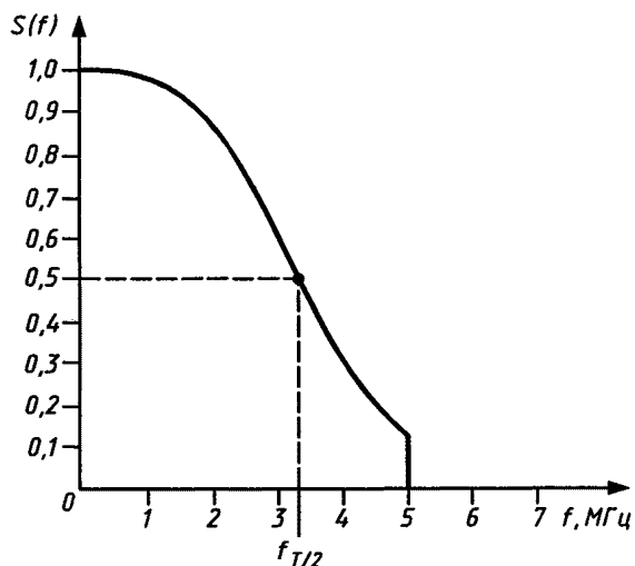
Рисунок 1 — Спектральная плотность импульса, соответствующего элементу цифрового сигнала
