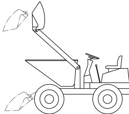
Рисунок 22 — Загрузка вспомогательным ковшом
