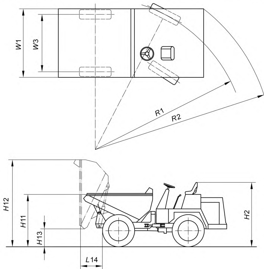
Рисунок 27 — Размеры четырехколесного мини-самосвала
