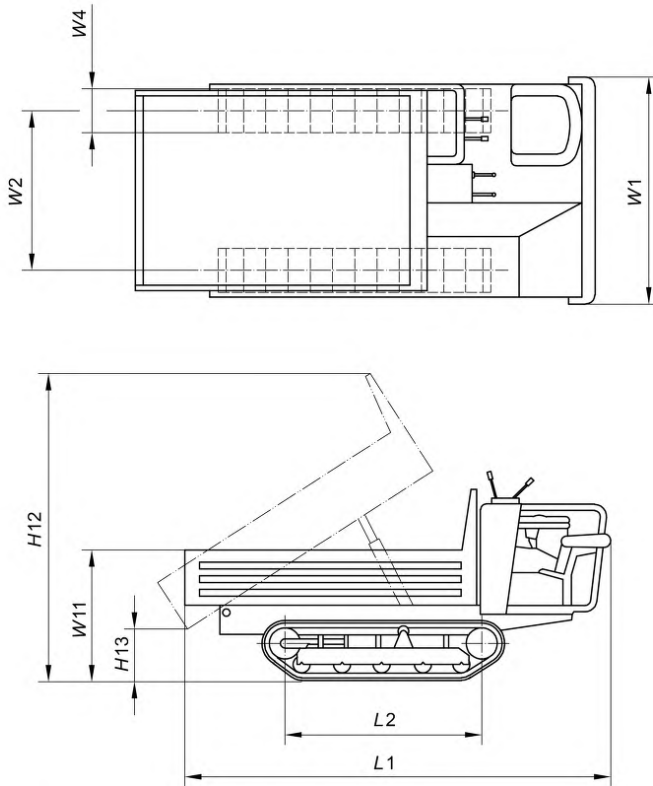
Рисунок 29 — Размеры гусеничного мини-самосвала. Рабочее место оператора сзади
