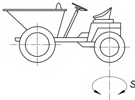
Рисунок 10 — Управление задними колесами
