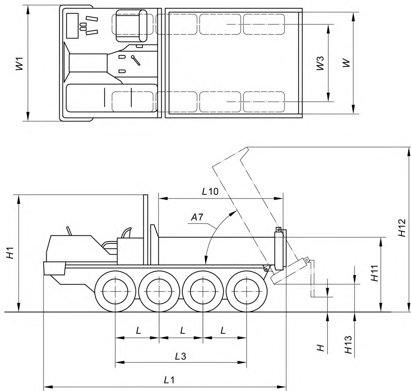
Рисунок 28 — Размеры восьмиколесного мини-самосвала
