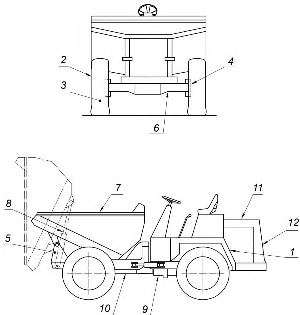
1 — крыло; 2 — колесо; 3 — шина; 4 — тормозная система; 5 — ось и корпус шарнира; 6 — ось (оси); 7 — кузов; 8 — гидроцилиндр; 9 — трансмиссия; 10 — основная рама; 11 — капот; 12 — энергетическая установка
