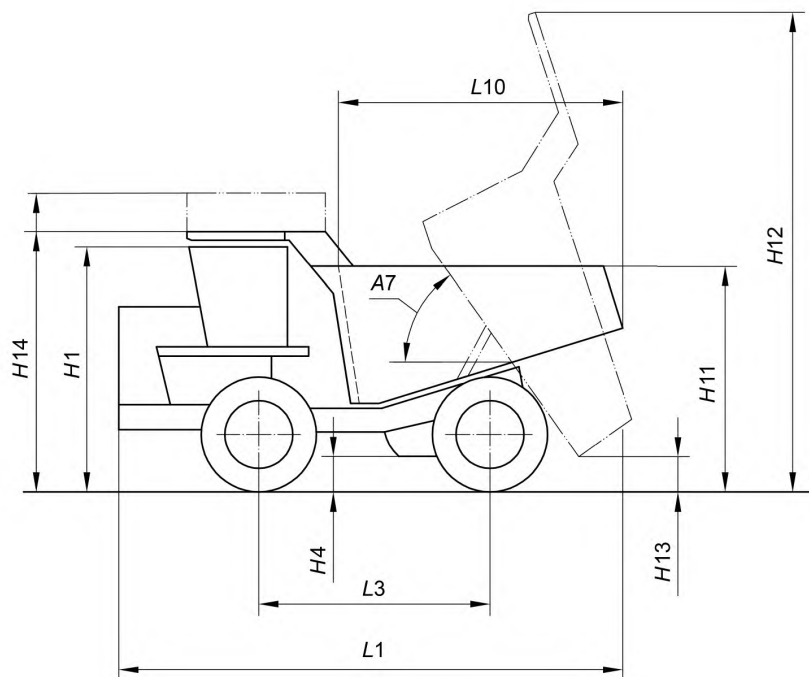
а) Жесткая рама
