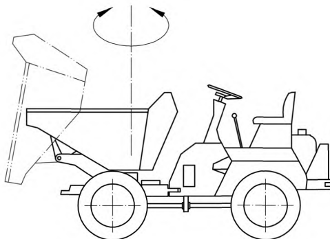
Рисунок 5 — Поворотная разгрузка
