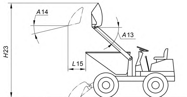
Рисунок 31 — Размеры мини-самосвала с самозагрузкой
