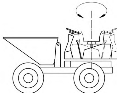
Рисунок 25 — Реверсивное рабочее место оператора
