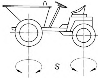
Рисунок 11 — Управление всеми колесами
