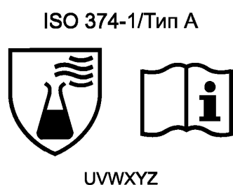
Рисунок 2 — Маркировка перчаток типа А
