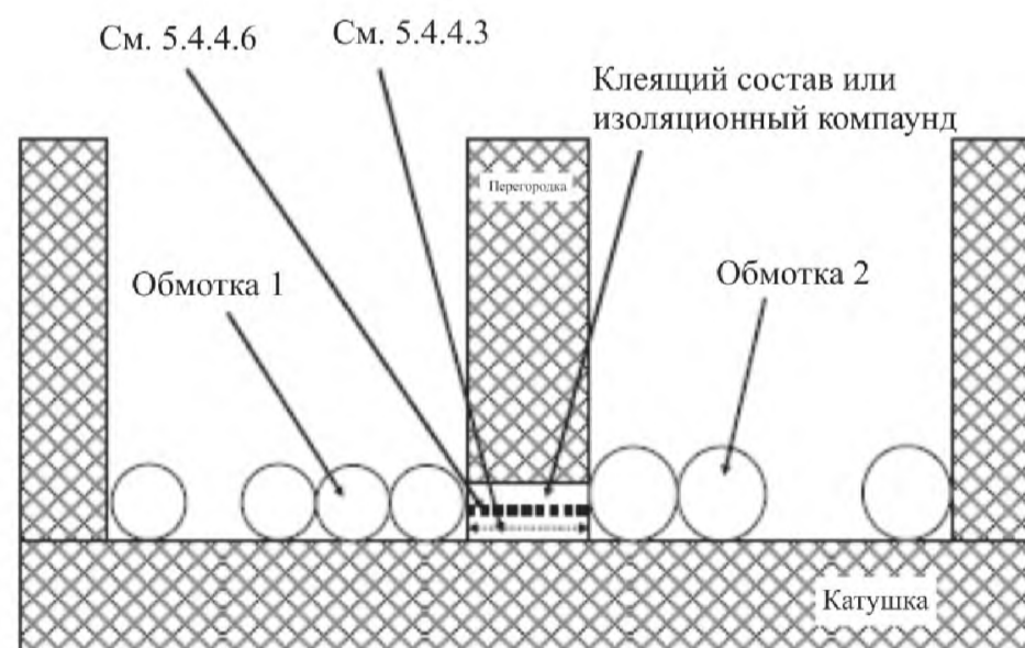
Рисунок О.16 — Секционированная катушка
