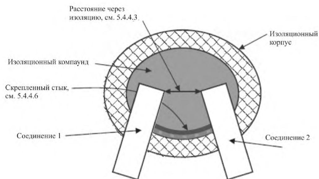
Рисунок О.15 — Устройство, заполненное изоляционным компаундом
