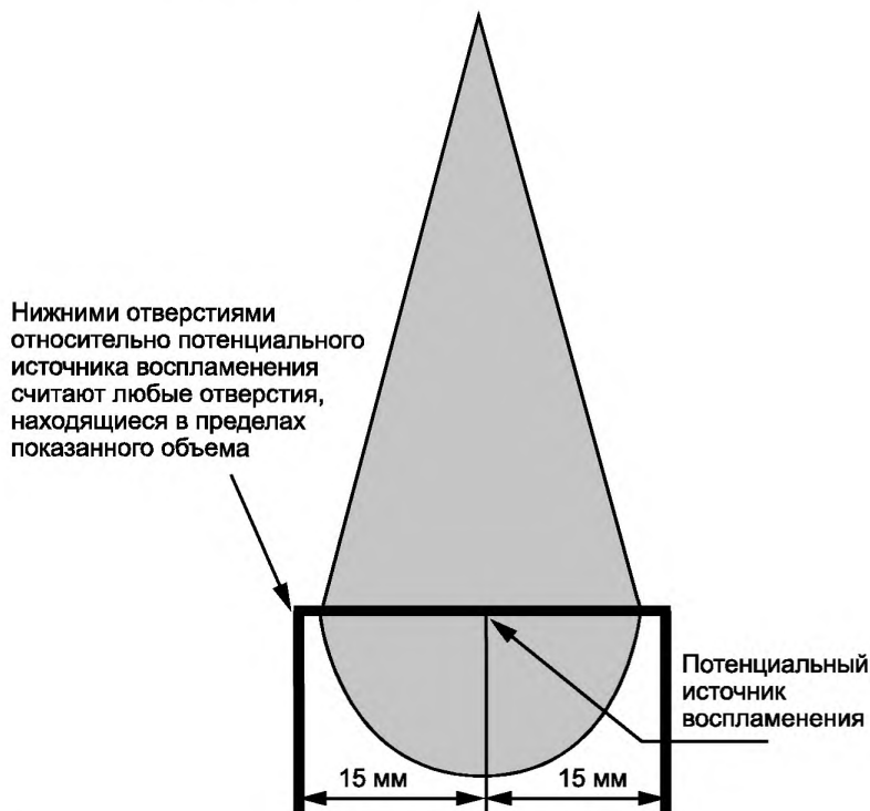
Рисунок 46 — Нижние отверстия
