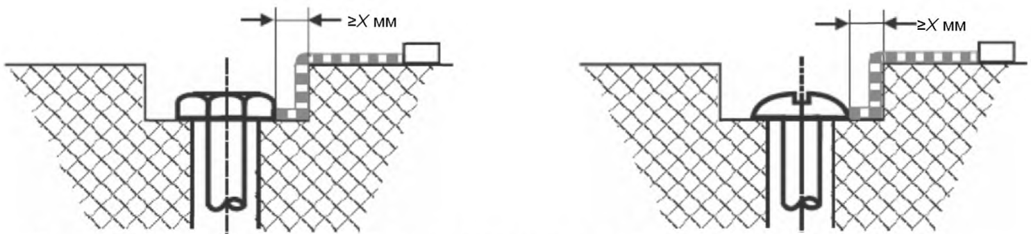
Рисунок O.10 — Большое углубление
