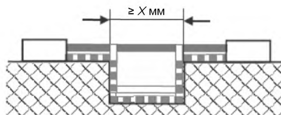
Рисунок О.1 — Узкая канавка
