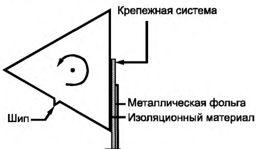
Рисунок 33 — Начальное положение оправки
