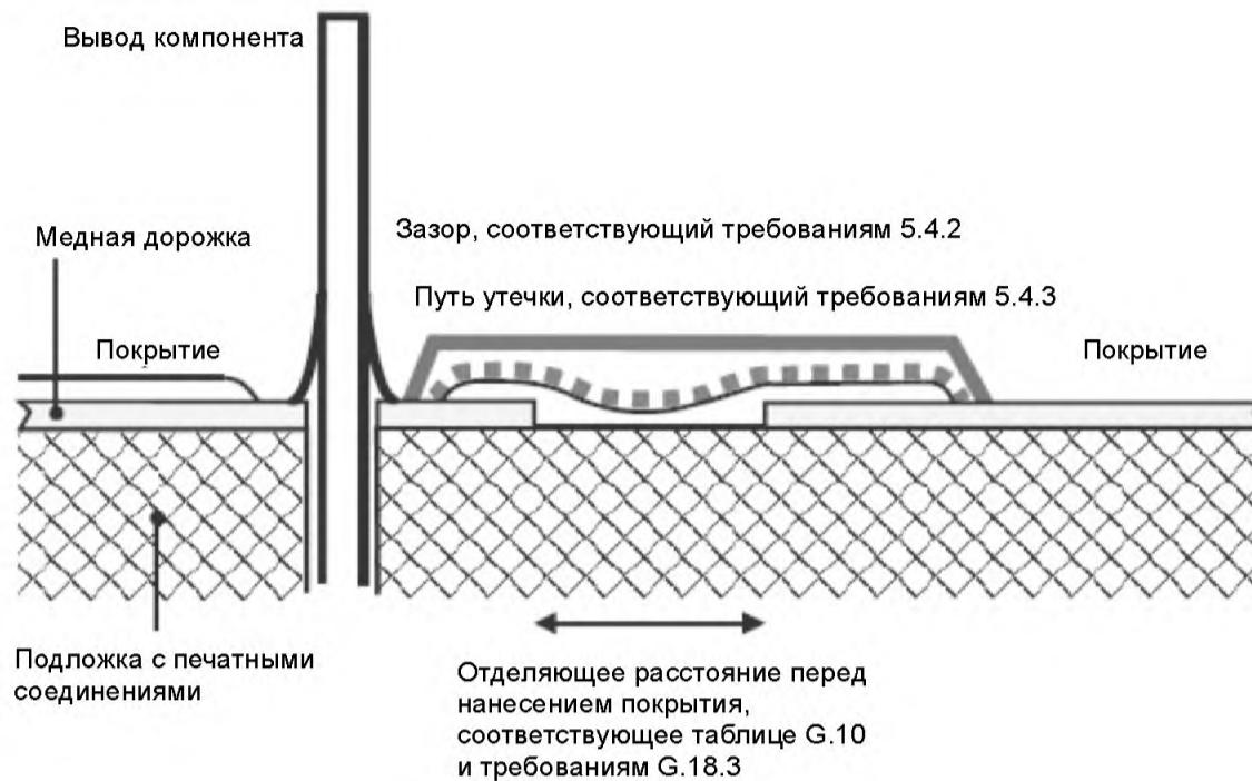
Рисунок O.12 — Покрытие поверх печатного монтажа
