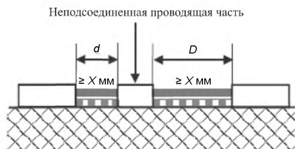
Рисунок О.3 — V-образная канавка
