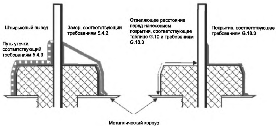
Рисунок O.11 — Покрытие выводов
