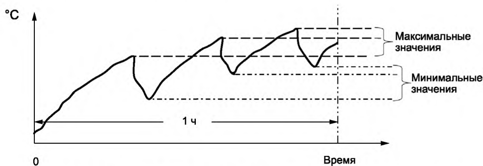
Рисунок G.1 — Определение среднеарифметического значения температуры
