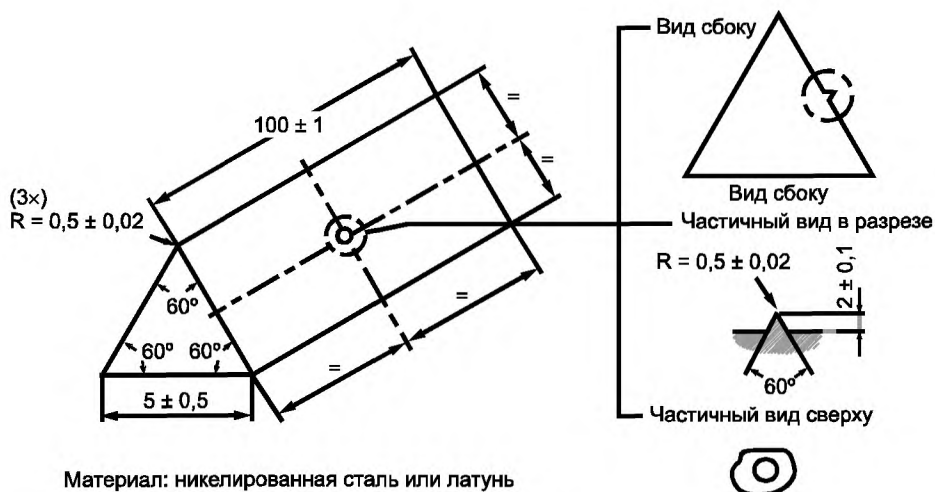
Рисунок 32 — Оправка
