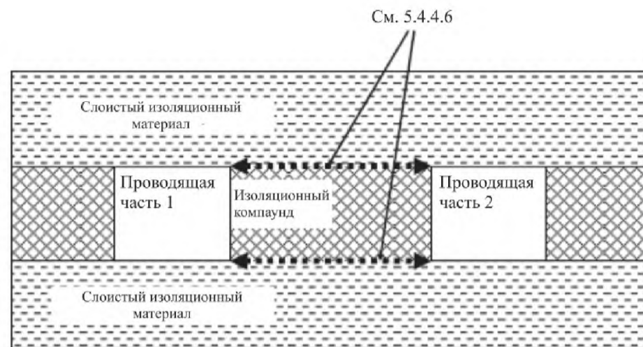
Рисунок О.14 — Скрепленные стыки в многослойных печатных платах
