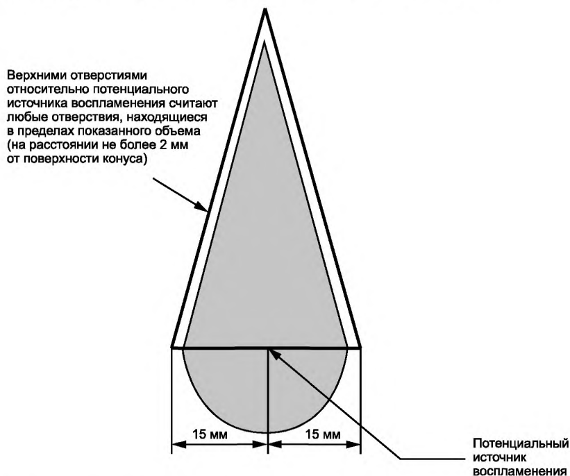
Рисунок 45 — Верхние отверстия
