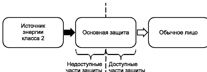
Рисунок 20 — Изображение доступных и недоступных частей основной защиты
