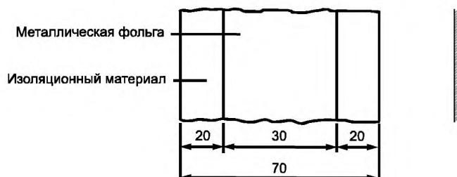
Рисунок 35 — Расположение металлической фольги на изоляционном материале
