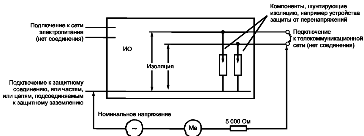
Рисунок 37 — Испытание разделения между телекоммуникационной сетью и землей
