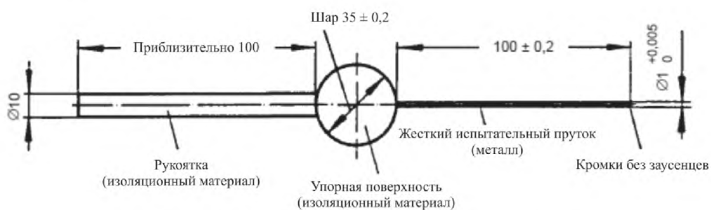
Рисунок V.5 — Щуп для испытания клемм
