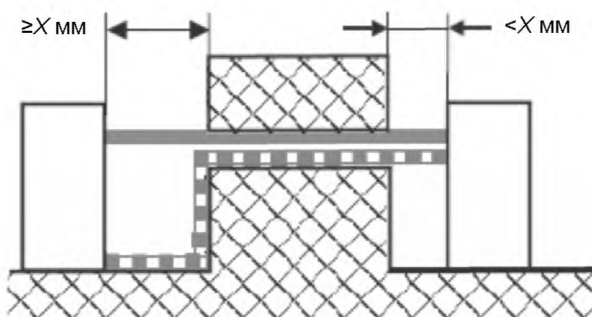
Рисунок О.7 — Нескрепленный стык с широкой канавкой
