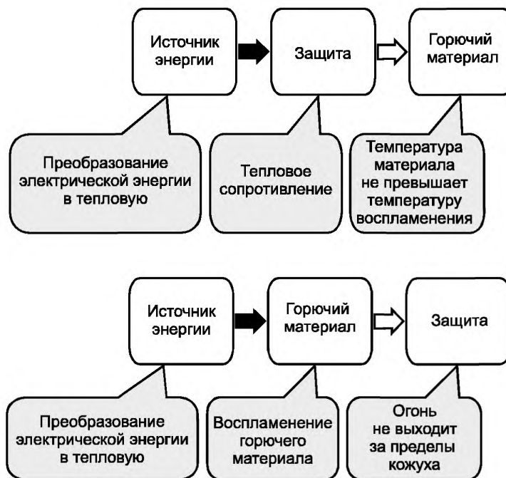
Рисунок 6 — Модели защиты от возгораний
