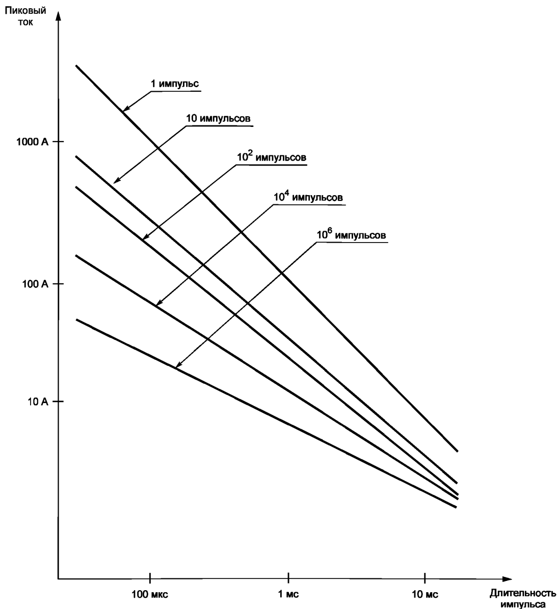
Рисунок 2 — Пример максимального пикового тока
