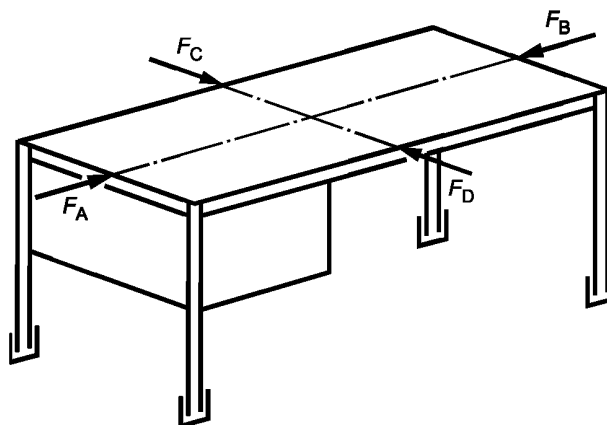
Рисунок А.1 — Определение механической прочности конструкции
