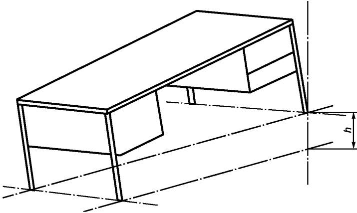
Рисунок 4 — Испытание падением
