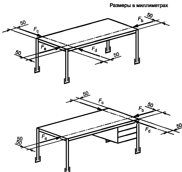
Рисунок 2 — Определение долговечности под действием горизонтальной нагрузки
