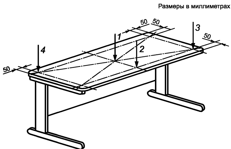
Рисунок 1 — Определение прочности под действием вертикальной нагрузки
