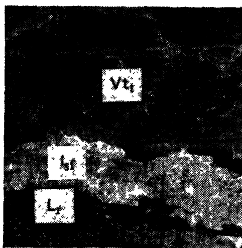
Vt_t — телинит; I_{sf} — semifюзинит; L_r — резинит
