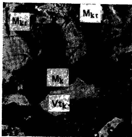
Vt_k — коллинит; M_k — карбонаты (кальцит); M_{kr} — кварц
