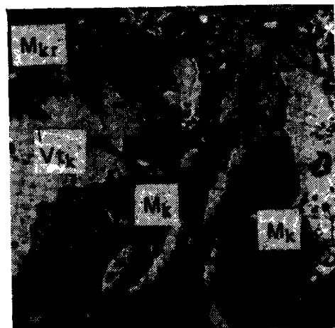
Vt_k — коллинит; M_r — карбонаты; M_{kr} — кварц
