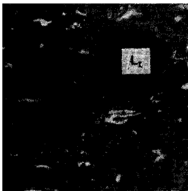
L_r — резинит Рисунок 12 — Масляная иммерсия 665×
