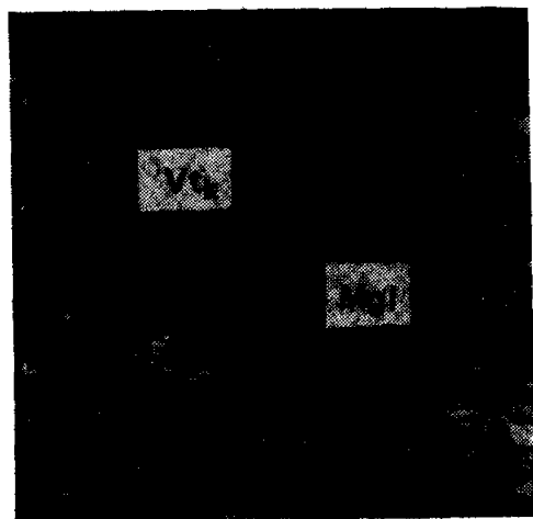
Vt_k — коллинит; M_{gl} — глинистые минералы
