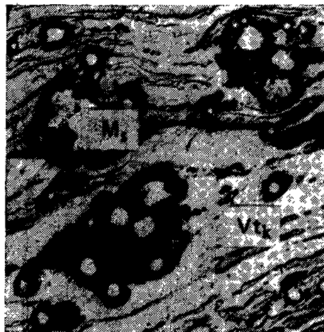
Vt_k — коллинит; M_s — сульфиды железа
