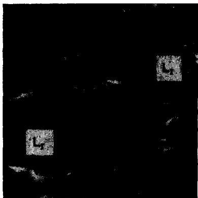
L_r — резинит Рисунок 11 — Масляная иммерсия 665×
