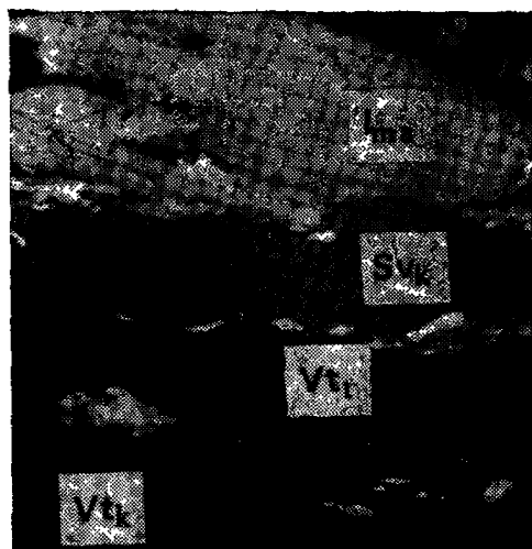
Vt_k — коллинит; Vt_t — телинит; Sv_k — семиколлинит; I_{ma} — макринит
