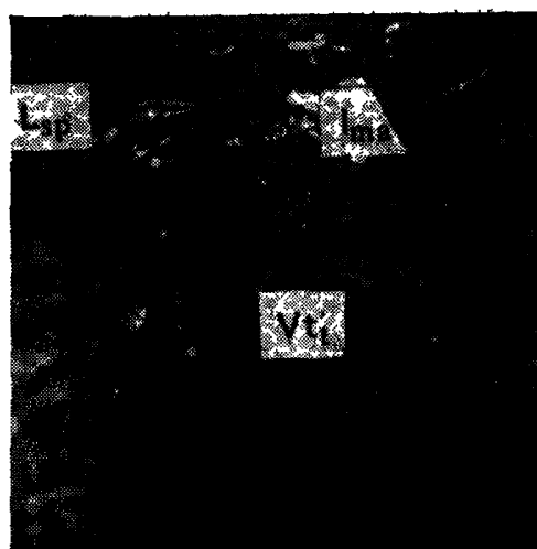
Vt_t — телинит; I_{ma} — макринит; L_{sp} — споринит
