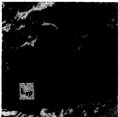
L_{sp} — споринит Рисунок 9 — Масляная иммерсия 400×
