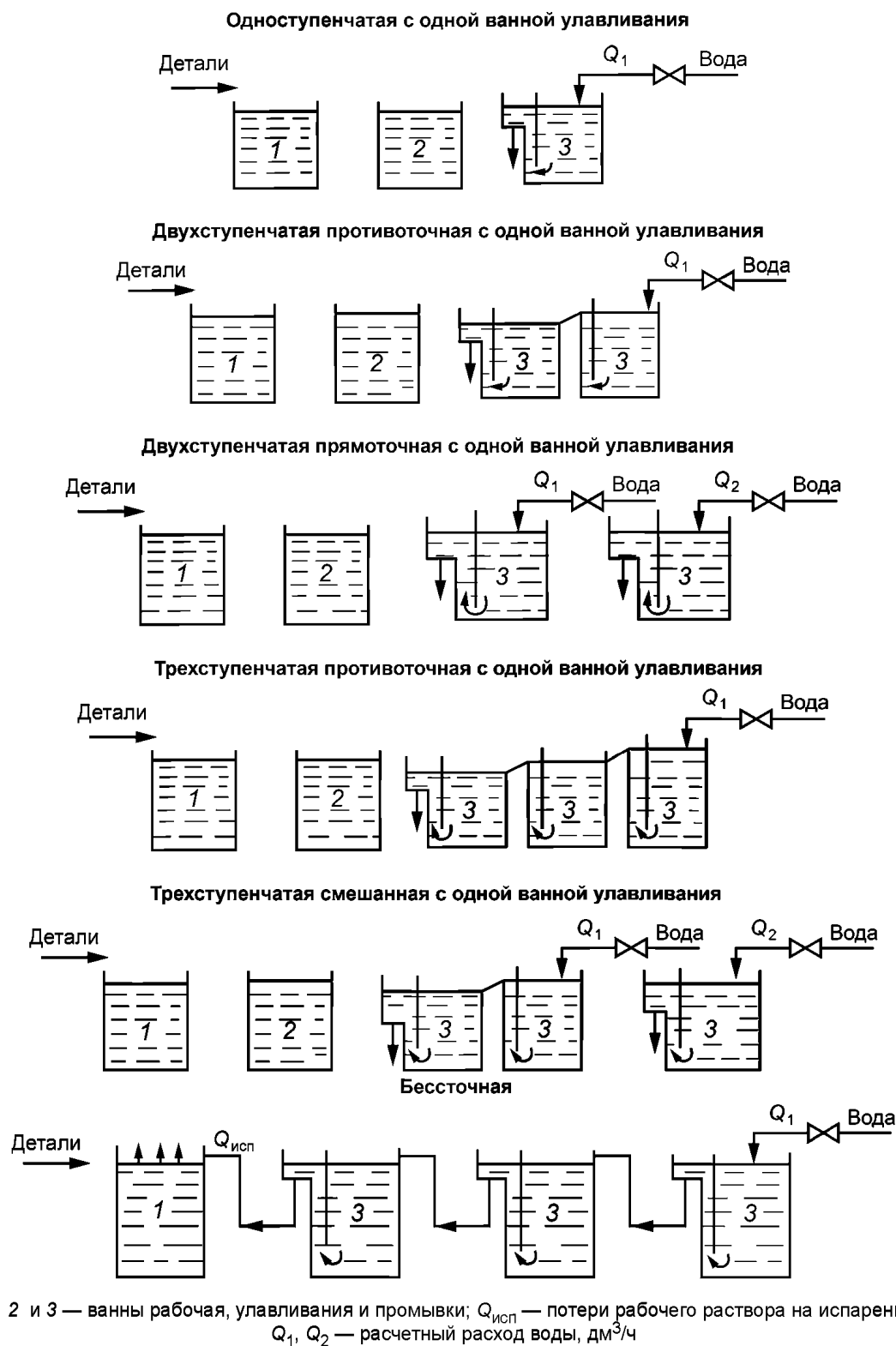
Рисунок 2 — Схемы промывок
