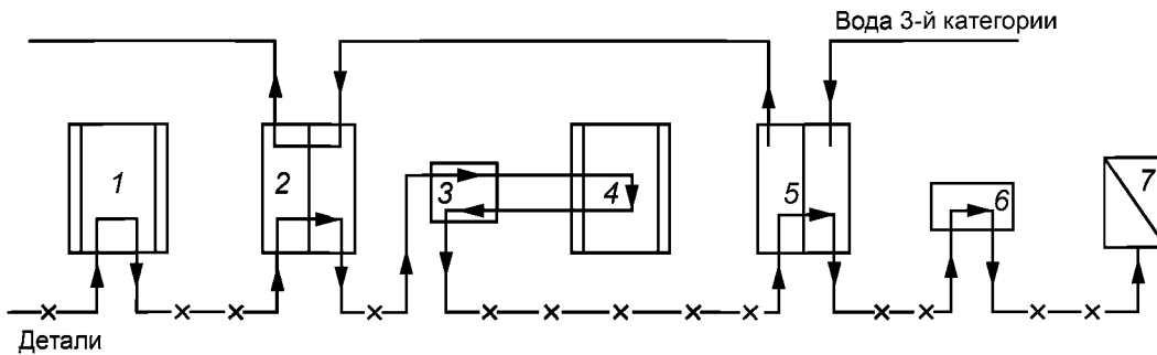
1 — ванна активации; 2, 5 — ванны промывки; 3 — ванна улавливания с водой 3-й категории; 4 — ванна нанесения покрытий; 6 — обдув сжатым воздухом или центрифугирование; 7 — сушка (термосушка)
