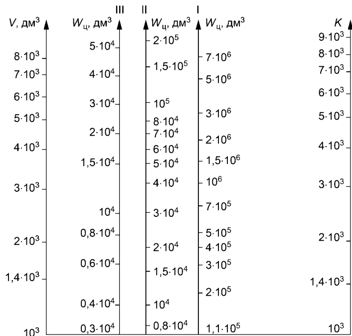
Рисунок 3 — Расчет объема воды для противоточных схем промывок
