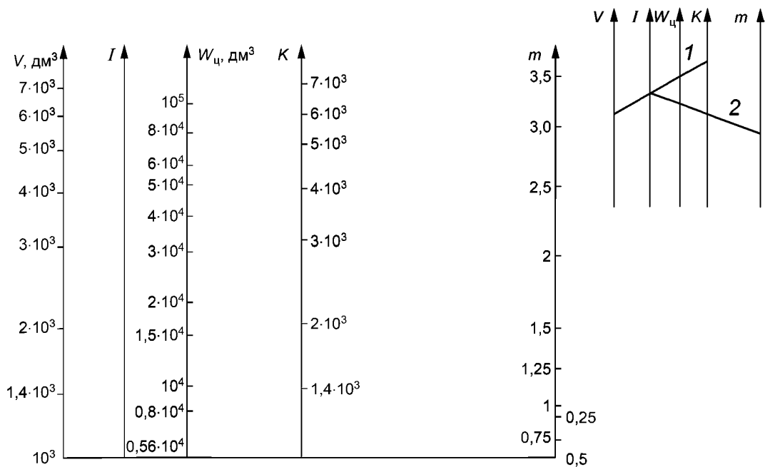
Рисунок 5 — Расчет объема воды при трехступенчатой смешанной промывке
