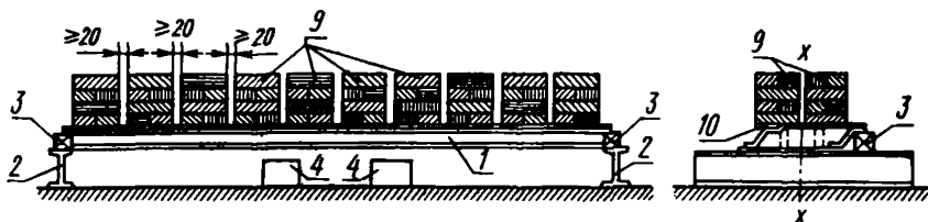
1—испытуемая плита; 2—опоры; 3—подпорки под верхнюю полку плиты; 4—предохранительные стойки; 9—тарированные грузы; 10—прокладка под грузами.
