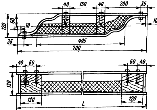
Поперечный и продольный разрезы рядовой плиты
