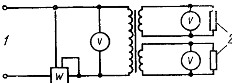
1 — источник питания; 2 — заменяющие резисторы
