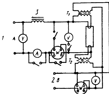
1, 2 — источники питания А и В, 3 — образцовый балласт
