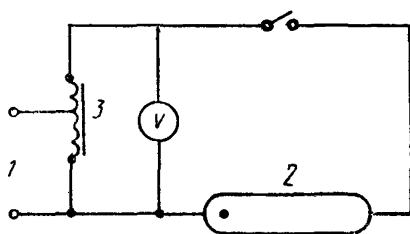
1 — источник питания; 2 — лампа; 3 — балласт
