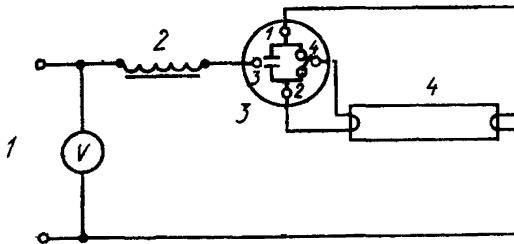
1 — источник питания, 2 — балласт, 3 — стартер, 4 — лампа
