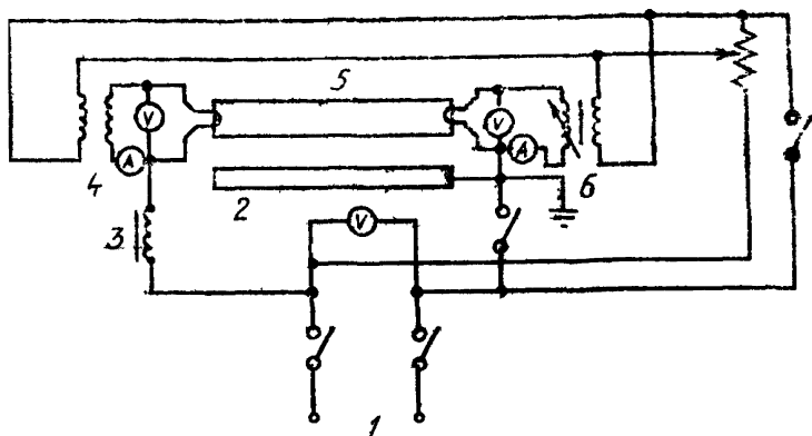
1 — источник питания; 2 — зажигающая полоса; 3 — балласт; 4, 6 — трансформаторы; 5 — лампа
