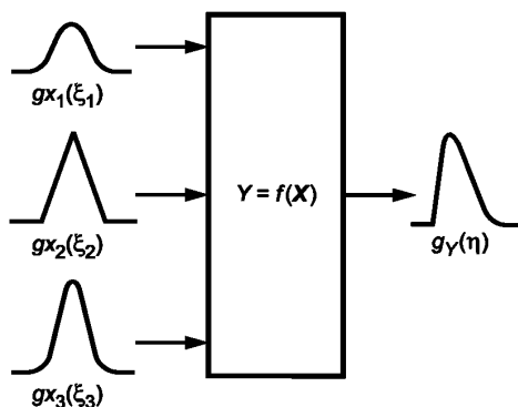
Рисунок 2 — Трансформирование распределений трех ( N = 3 ) независимых входных величин
