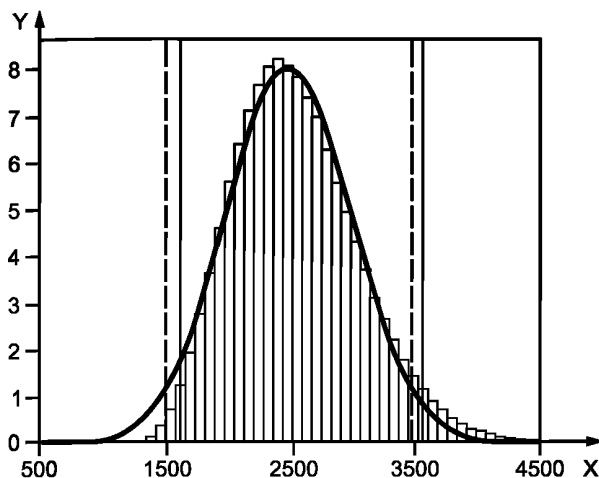
X — отклонение \delta Y коэффициента рассогласования от единицы (умноженное на 10^6 ), Y — плотность распределения вероятностей (умноженная на 10^4 )
