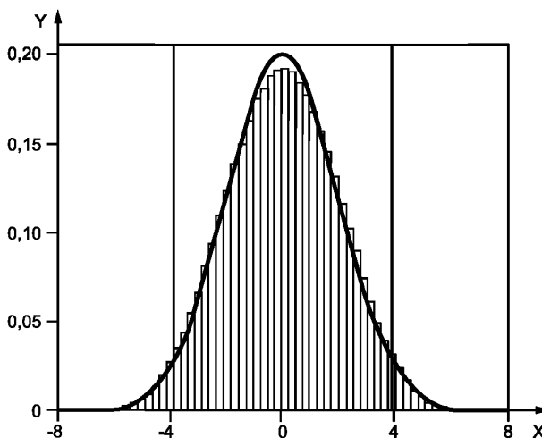
X — величина (безразмерная), Y — плотность распределения вероятностей
