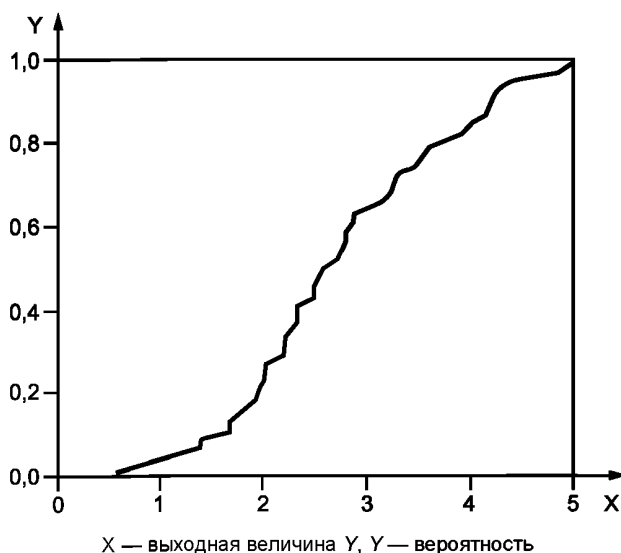
Рисунок D.1 — Аппроксимация \tilde{G}_Y(\eta) функции распределения G_Y(\eta)
