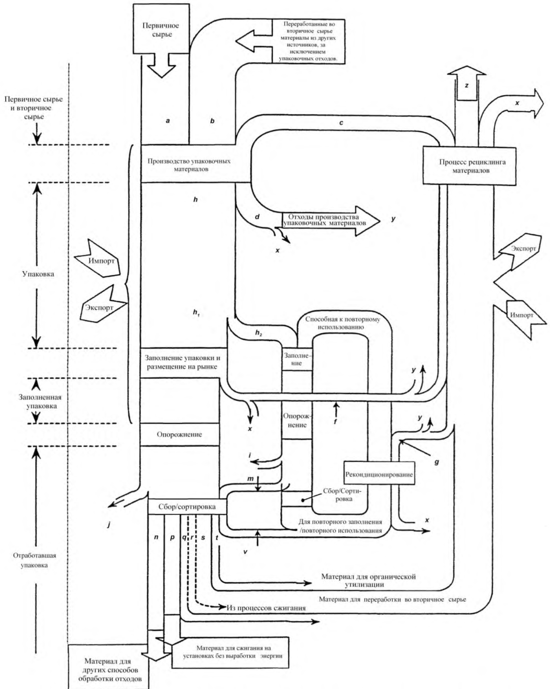
Рисунок А.1 – Потoki для переработки упаковки в качестве вторичных материальных ресурсов
