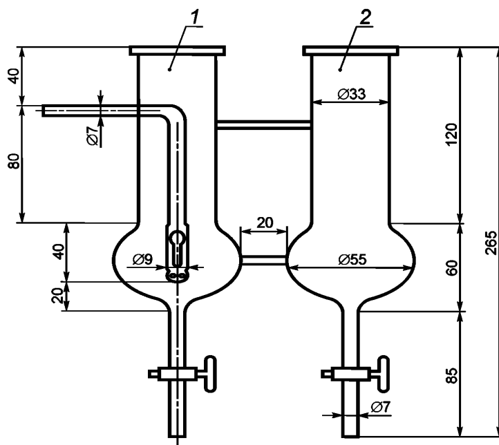
Рисунок 2 — Устройство поглотительного сосуда
