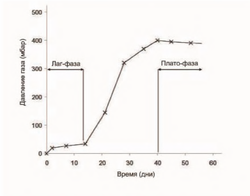
Рисунок В.1 – Пример кривой биоразложения
