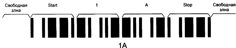
Рисунок 1. Символ Code 39
