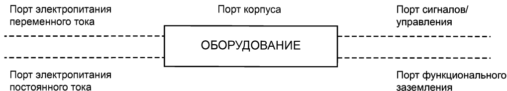
Рисунок 1 — Примеры портов
