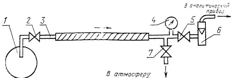
1—заводской трубопровод; 2, 5, 7—клапаны; 3—трубопровод для подачи газа к месту анализа; 4—манометр; 6—ротаметр, реометр или другой газовый счетчик
