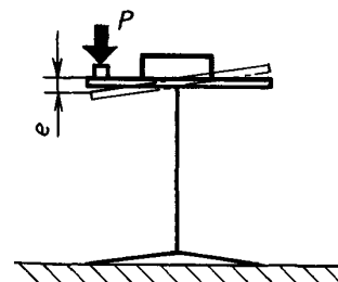
P — нагрузка; e — деформация
