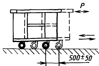
P — нагрузка
