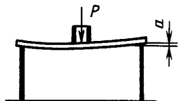
P — нагрузка; a — прогиб
