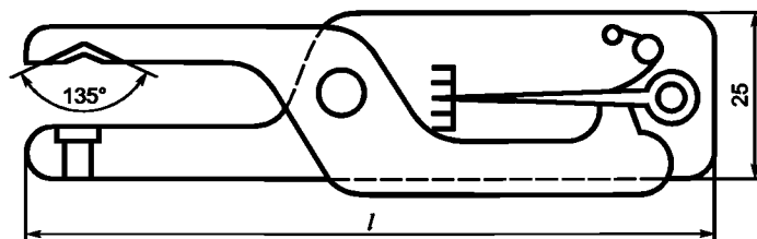
Рисунок В.1 — Шаблон для измерений
