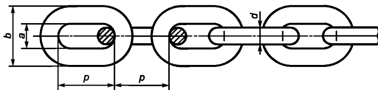
Рисунок 1 — Калиброванная цепь
