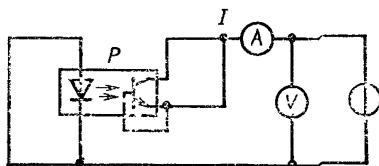
P — измеряемая фотопара
