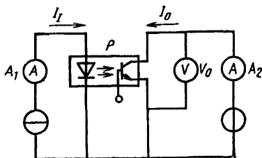
Принципиальная схема
