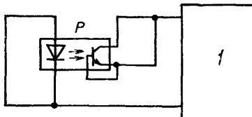
P — измеряемая фотопара I — измеритель емкости
