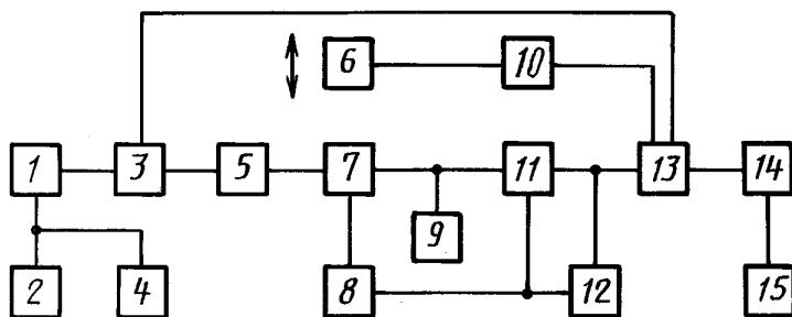
1 — осветитель монохроматора; 2 — источник питания осветителя; 3 — световой затвор с устройством управления; 4 — вольтметр контроля напряжения питания осветителя; 5 — устройство выделения монохроматического излучения; 6 — опорный приемник; 7 — прибор; 8 — синхрогенератор или блок задания электрического режима; 9 — резистор нагрузки ампервольтметра для измерения выходного сигнала опорного приемника; 11 — усилитель; 12 — устройство отображения выходного сигнала; 13 — устройство измерения; 14 — ЭВМ; 15 — графопостроитель
