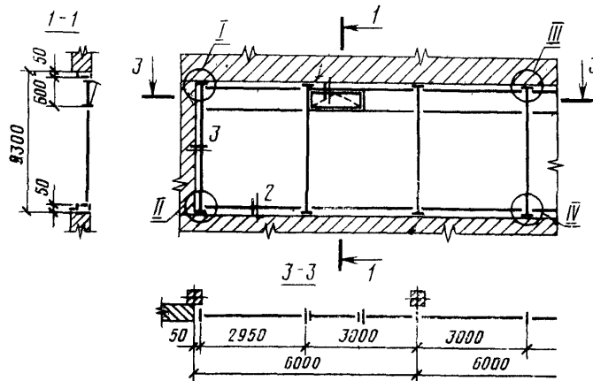
Схема установки витражей верхнего и типовых этажей
