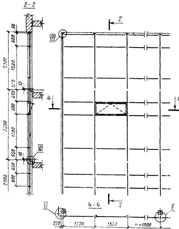
Схема установки витражей верхнего и типовых этажей
