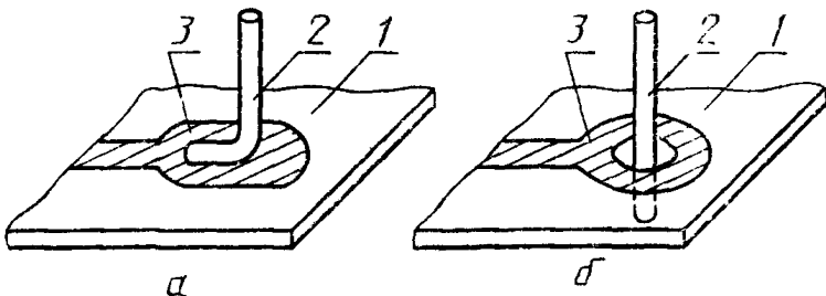
1—плата 2—проволока 3—контактная площадка (металлизированное отверстие)
