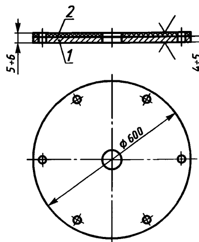
1 — стальной диск; 2 — испытуемое покрытие
