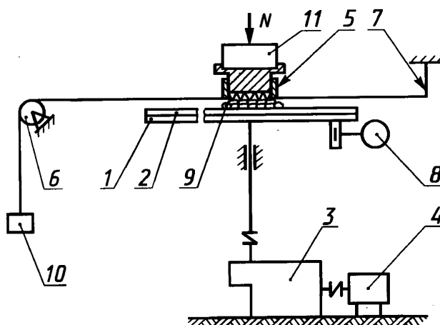
1 — опорный подвижный диск; 2 — образец; 3 — редуктор; 4 — приводной электродвигатель; 5 — цилиндрический короб; 6 — блок тарировочного устройства; 7 — тензобалка; 8 — тахометр; 9 — испытываемая волокнистая масса; 10 — груз; 11 — тарировочный груз
