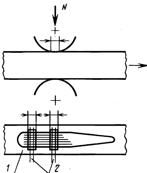
1 — контур поверхности контакта; 2 — трассы профилографирования
