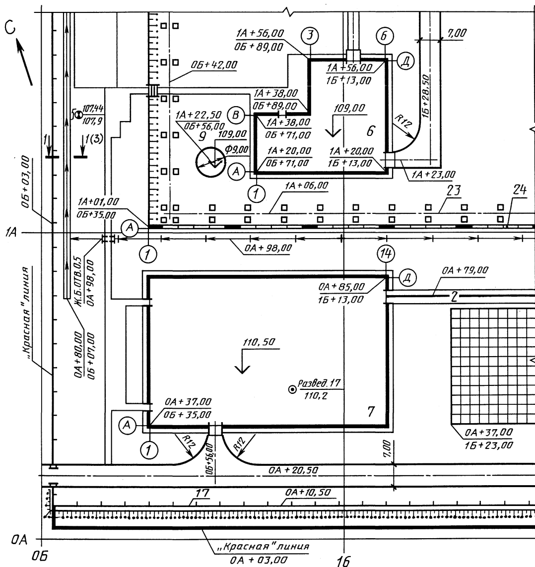
Пример оформления разбивочного плана
