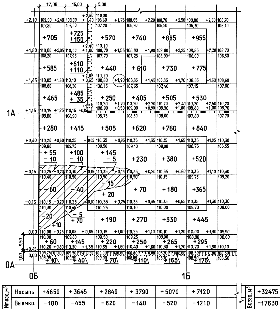
Пример оформления плана земляных масс
