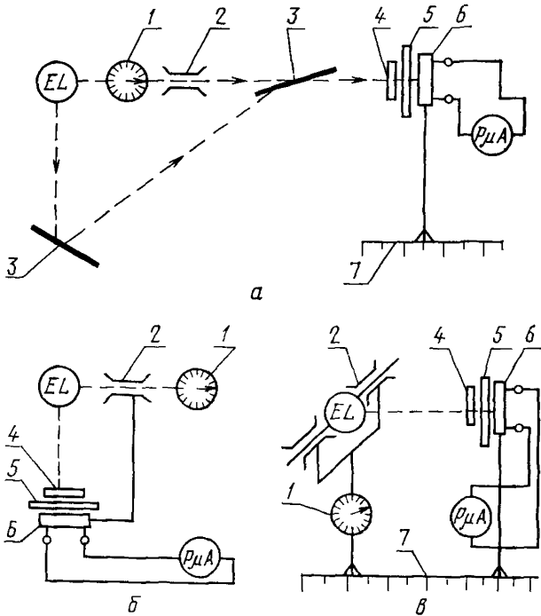
EL—измеряемая лампа; 1—линза; 2—ось вращения; 3—зеркала; 4—нейтральный светофильтр; 5—светорассеивающее стекло; 6—приемник излучения; 7—фотометрическая шкала, PμA—прибор, измеряющий фототок
