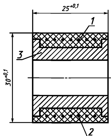
1 — покрытие из токопроводящей резины; 2 — проводочный бандаж; 3 — латунная втулка
