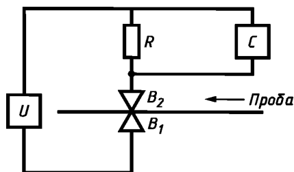
C — регистрирующее устройство; U — источник постоянного напряжения; B 1 , B 2 — контактные валики; R — резистор
