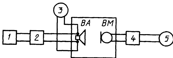
1 – генератор ГНИ; 2 – усилитель мощности У1; 3 – электронный вольтметр; 4 – микрофонный усилитель УМ; 5 – измеритель нелинейных искажений ИНИ; BA – контролируемый громкоговоритель; BM – измерительный микрофон
