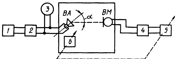
1 – генератор ГНИ; 2 – усилитель мощности У1; 3 – электронный вольтметр; 4 – микрофонный усилитель УМ; 5 – регистрирующее устройство; 6 – поворотный стол; ВА – контролируемый громкоговоритель; ВМ – измерительный микрофон
