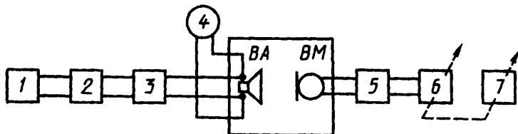
1 – генератор розового шума ГШН; 2 – фильтр ФЭД; 3 – усилитель У1; 4 – электронный вольтметр; 5 – микрофонный усилитель УМ; 6 – переключаемый третьоктавный узкополосный фильтр; 7 – регистрирующее устройство
