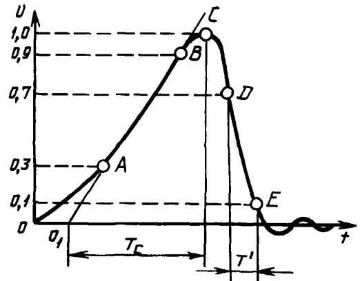
Рисунок 8 — Грозовой импульс, срезанный на фронте
