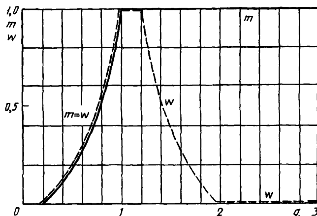
Рисунок 5 — Показатели степени m и w
