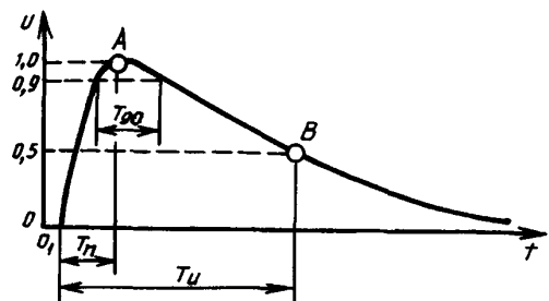
Рисунок 13 — Аperiodический коммутационный импульс
