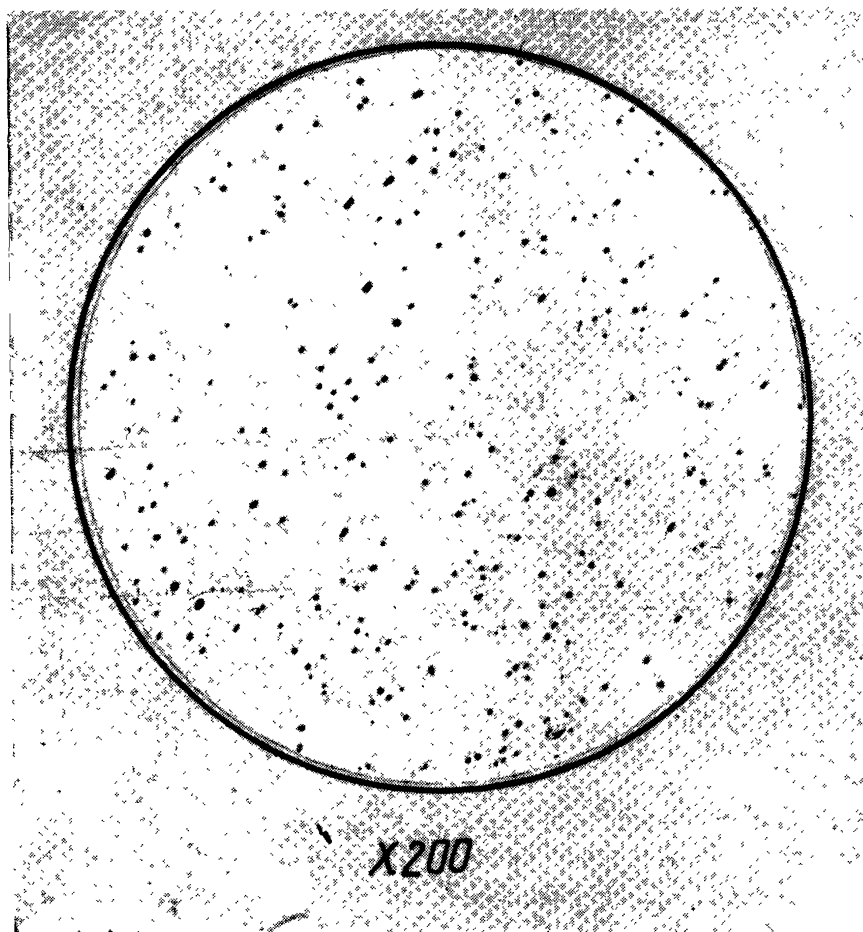
Черт. 2. Материал — деформированная медь, массовая доля кислорода — 0,03 %, освещение — рассеянный свет
