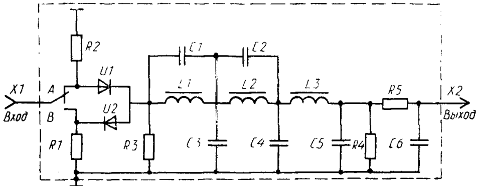
Схема детектора шума
