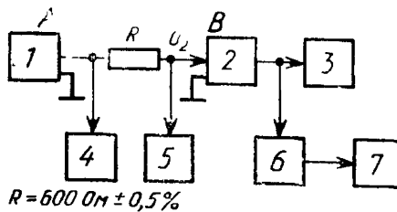
Схема измерения сопротивления низкочастотного входа передатчика
