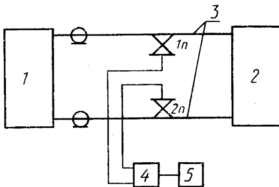
Схема подключения сумматора противофазных сигналов
