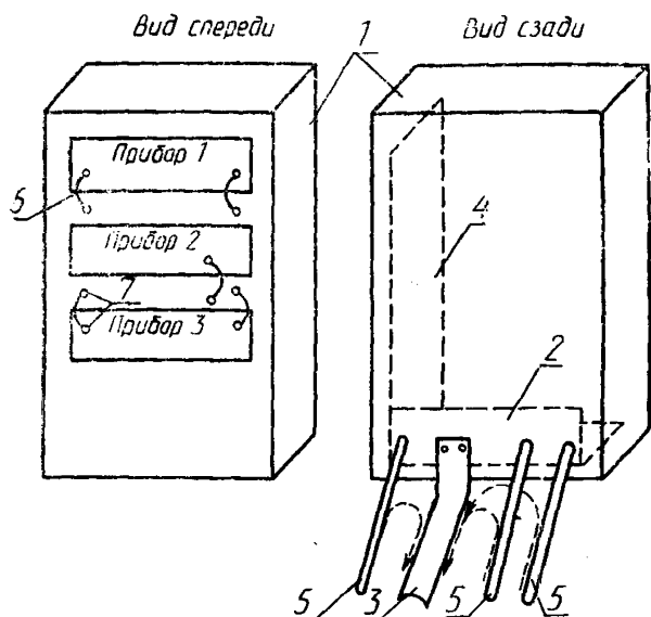
Средства групповой защиты измерительных приборов от радиопомех
