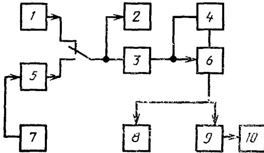
Схема измерения ширины контрольной полосы радиочастот
