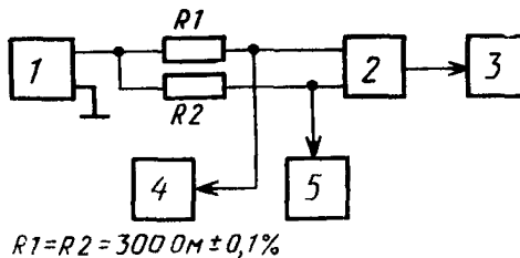
Схема измерения коэффициента асимметрии сопротивления низкочастотного входа передатчика с АМ
