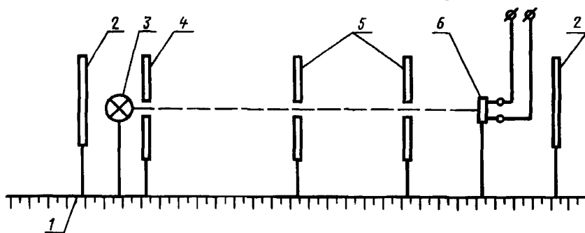
Схема градуировки светоизмерительной аппаратуры
