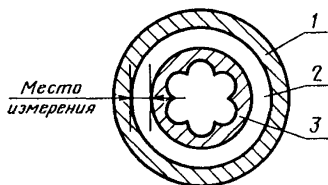
1 — оболочка, 2 — промежуточная зона, 3 — изоляция
