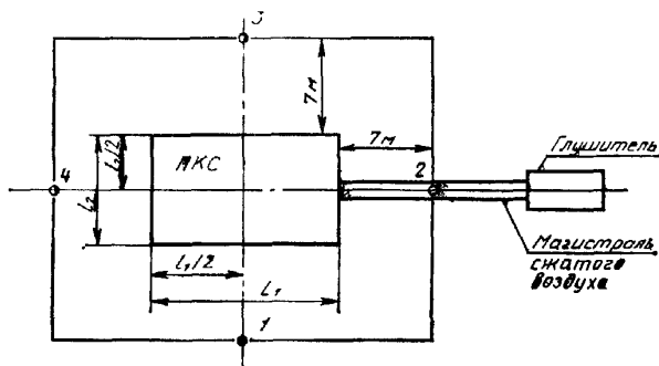
1—4 — точки измерения шума, L_1 и L_2 — длина и ширинагибающего источника шума параллелепипеда
