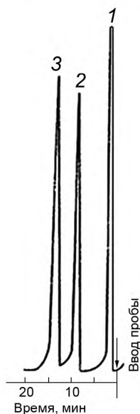
1 — растворитель, 2 — дециловый спирт, 3 — фенол
