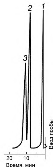
1 — растворитель, 2 — фенол, 3 — крезол
