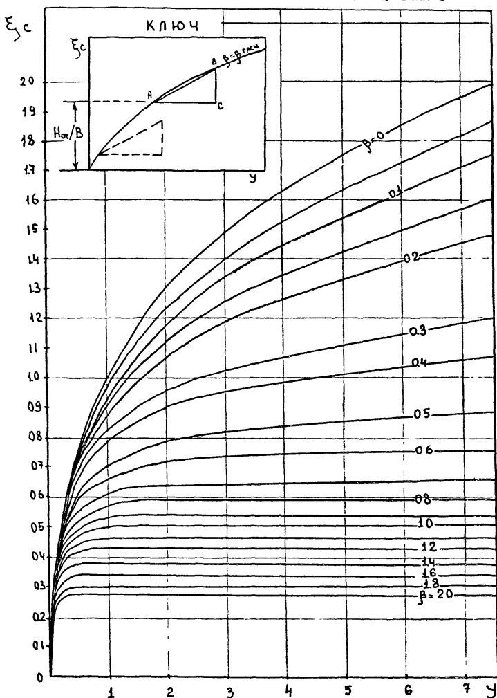
Рис. 3.1 Номограмма для определения \xi_c по H_{ст}/B Примечание: является известной номограммой \xi_c = f(J) СНиП П-18-76, в которой логарифмическая шкала J заменена равномерной и продлена до 7.
