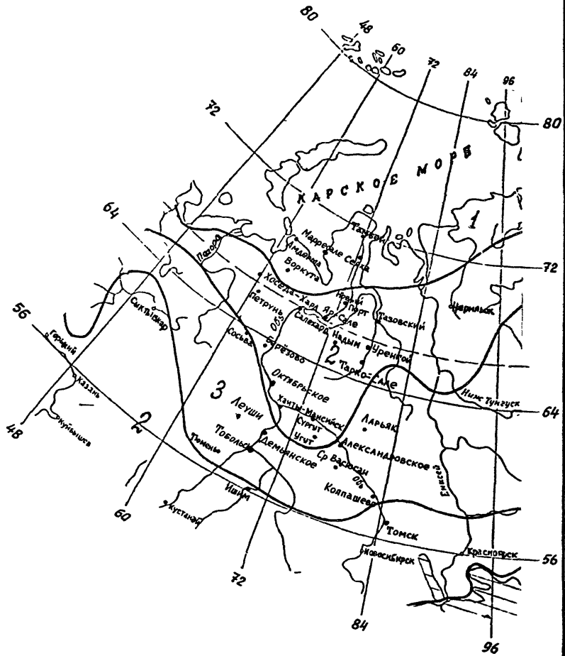
Рис.2.8. Схематическая карта распределения максимальных из средних скоростей ветра ( V м/с) по румбам за январь, повторяемость которых составляет \geq 16\%
