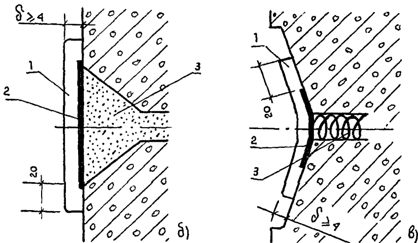
Рис. 1. Герметизация стыков тиokolовым герметиком: а) 1-3 — последовательность заполнения герметиком стыка; б) герметизация по жесткому основанию; в) герметизация по упругому основанию 1—герметик; 2—самоклеющаяся полимерная лента; 3—стык
