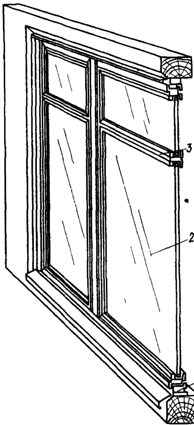
↑ Рис 2 Бесперелетное окно из профильного стекла
