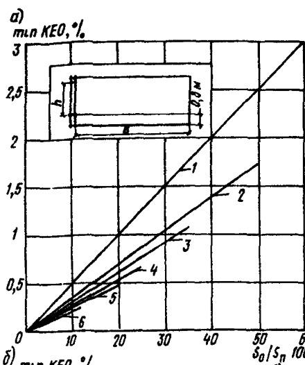
Рис 6 Графики для определения площади световых проемов при боковом освещении помещений при отношении
