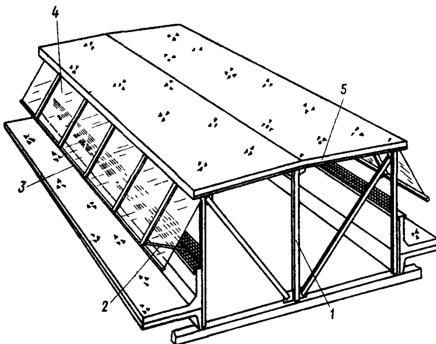
Рис 3 Светоаэрационный фонарь
