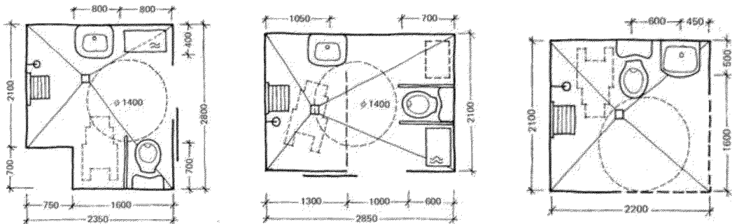
Рисунок 6.2.11 – Санузлы для МГН
