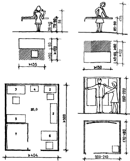
Рисунок 6.3.18 – Мастерская мелкого ремонта одежды:
