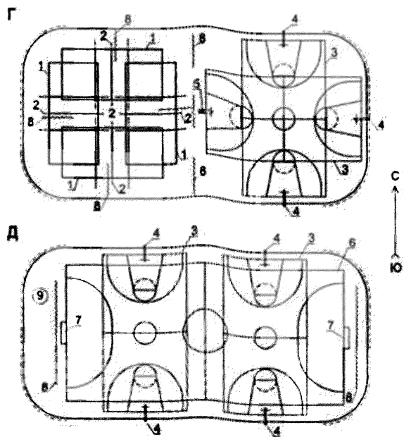
Рисунок 5.3 – Варианты компактной блокировки спортивных площадок: Г – для волейбола и баскетбола, Д – для мини-футбола, баскетбола, бадминтона и настольного тенниса
