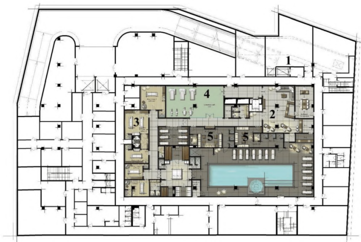
Рисунок 6.3.25 – Пример размещения бассейна в здании гостиницы «Хилтон Пречистенка», г. Москва: 1 – лифт на жилые этажи, 2 – бар у рецепции, 3 – комната отдыха занимающихся,
