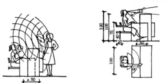
Рисунок 6.3.4 – Соответствие стойки оформления гигиеническим требованиям (слева) и требованиям работы и контакта с посетителями (справа)
