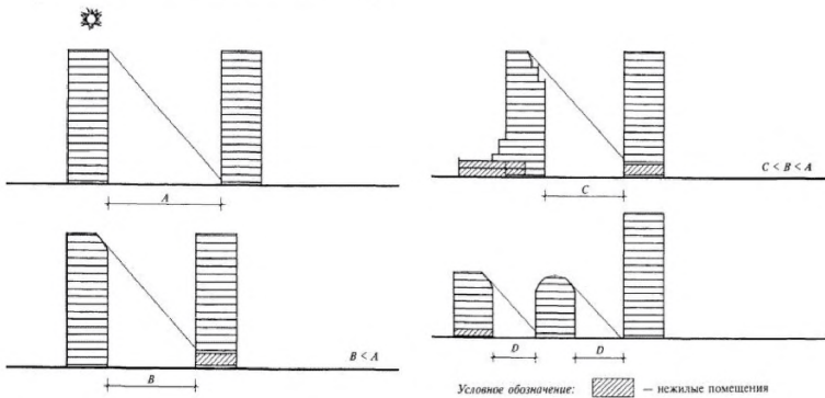
Рисунок 5.7 – Объемно-планировочные решения, позволяющие обеспечить необходимую инсоляцию зданиям, находящимся рядом с гостиницей, при высокой плотности застройки
