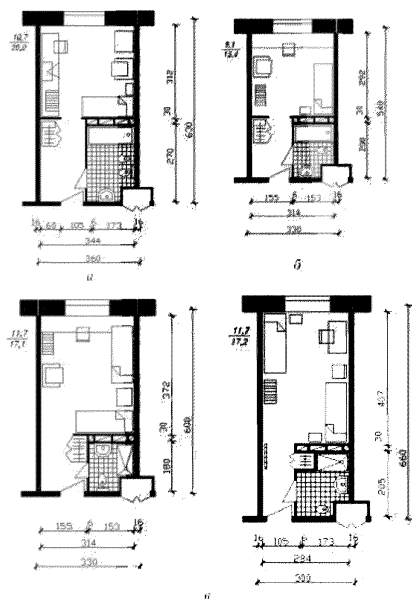
Рисунок 6.2.6 – Архитектурно-планировочные решения и примеры технологического оборудования жилых номеров разного уровня комфортности:
