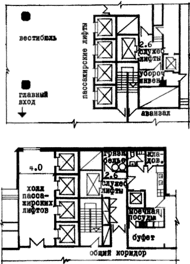
Рисунок 6.1.16 – Примеры планировочных решений лифтового холла в гостиницах большой вместимости
