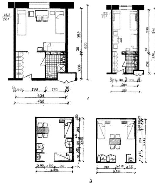
Рисунок 6.2.7 – Архитектурно-планировочные решения и примеры оборудования жилых номеров разного уровня комфортности:
