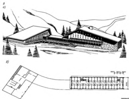
Рисунок 6.1.5 – Пример изоляции номеров от общественного блока
