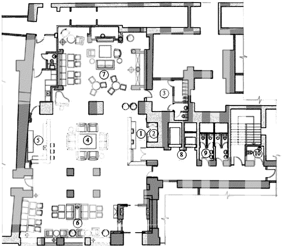
Рисунок 6.3.5 – Планировка вестибюля гостиницы:
