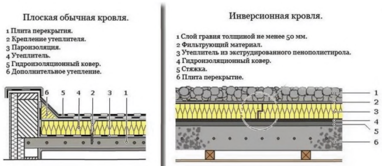
Рисунок 6.1.13 – Пример обычной и инверсионной кровли
