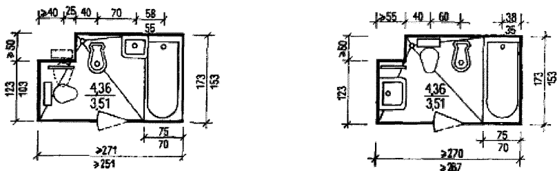
Рисунок 6.2.9 – Санузлы с ванной
