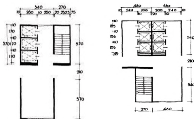
Рисунок 6.2.24 – Пример расположение поэтажного холла
